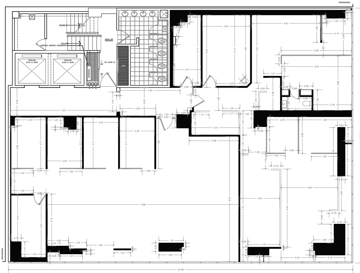
PLANTA SEXTO NIVEL (OFICINAS)
