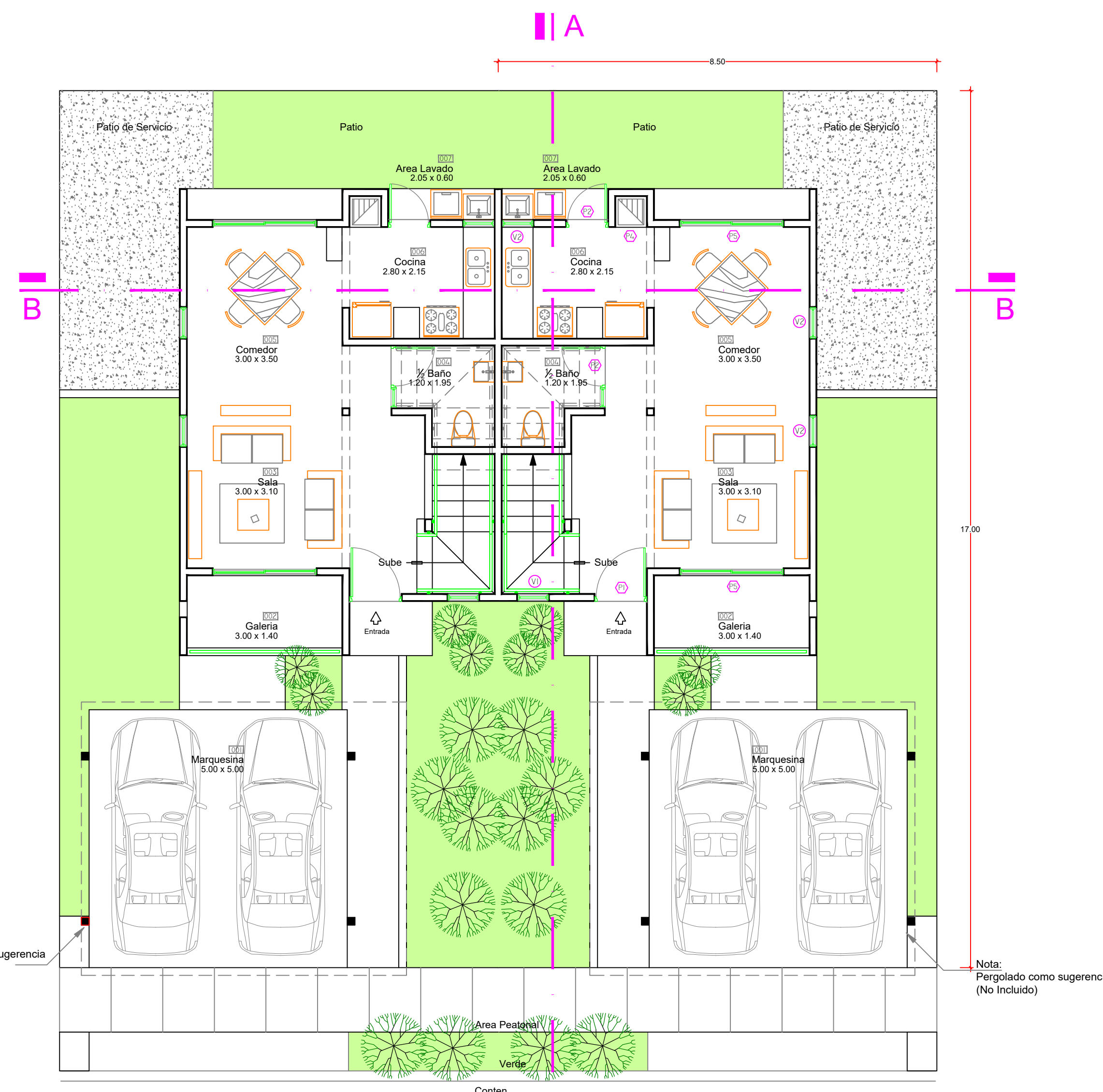
A 2.1 Planta Arquitectónica - 1er nivel Vivienda Duplex - Modelo C Area de Solar: 144.50 m 2 Area 1er Nivel: 52.87 m 2 ESC 1:75
