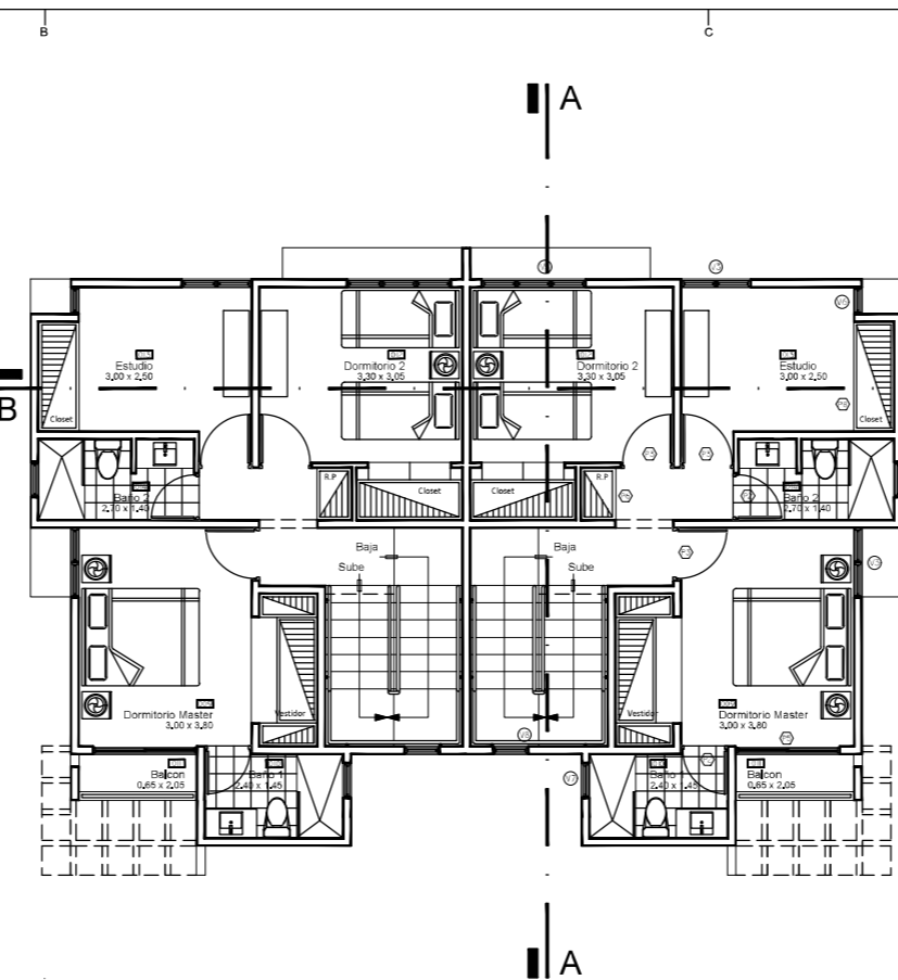
Planta Arquitectónica - 2do nivel Vivienda Duplex - Modelo A Área 2do Nivel: 64.10 m 2 ESC 1:75
