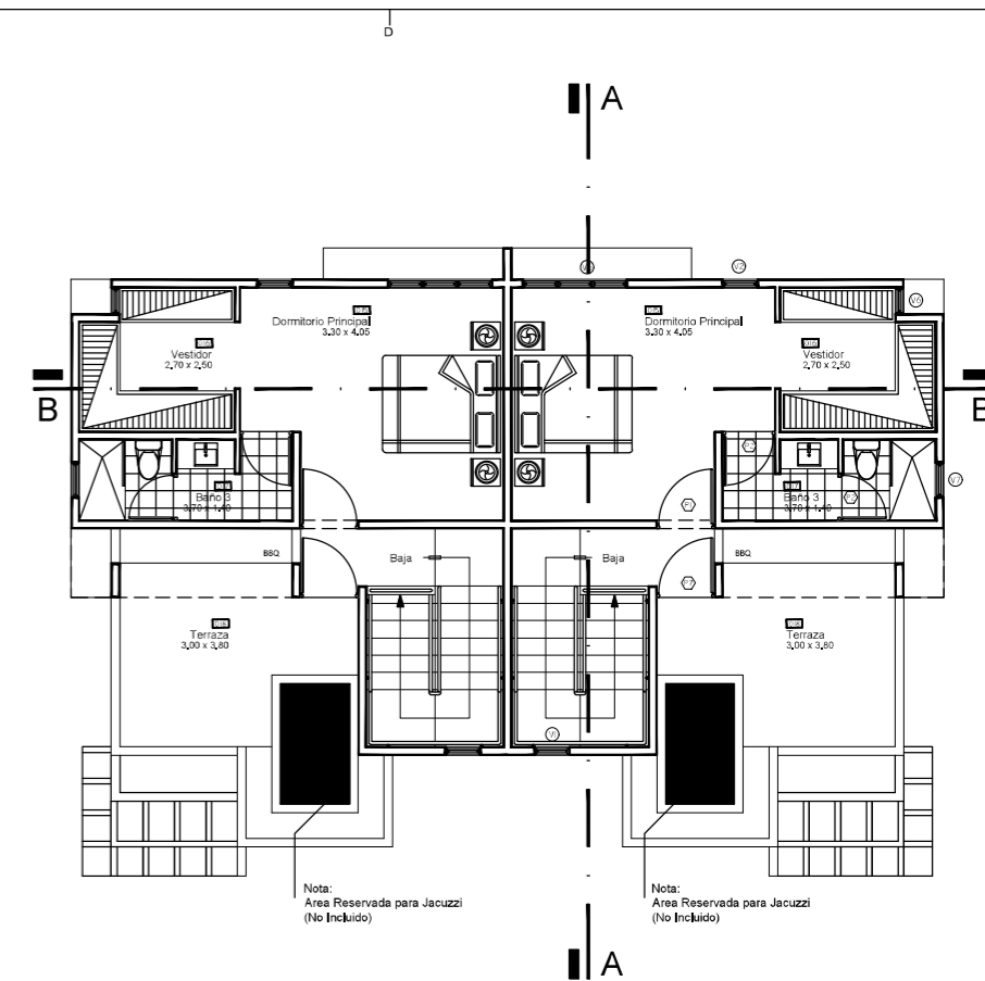
Planta Arquitectónica - 3er nivel Vivienda Duplex - Modelo A Área 3er Nivel: 64.10 m 2 ESC 1:75
