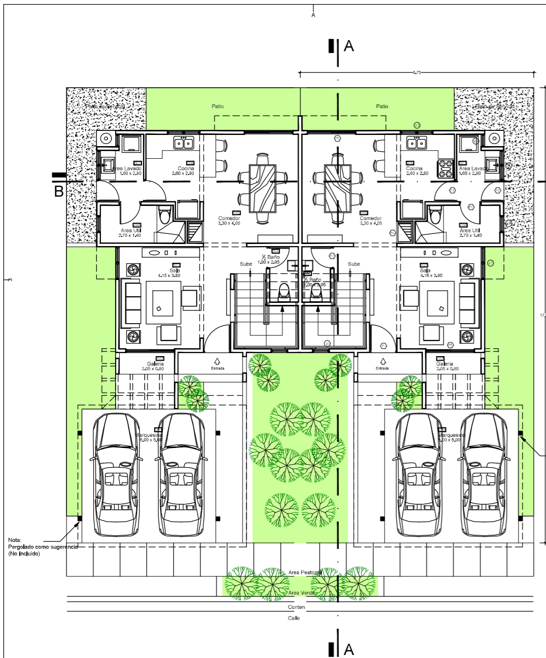
Planta Arquitectónica - 1er nivel Vivienda Duplex - Modelo A Área de Solar: 144.50 m 2 Área 1er Nivel: 62.42 m 2 ESC 1:75
