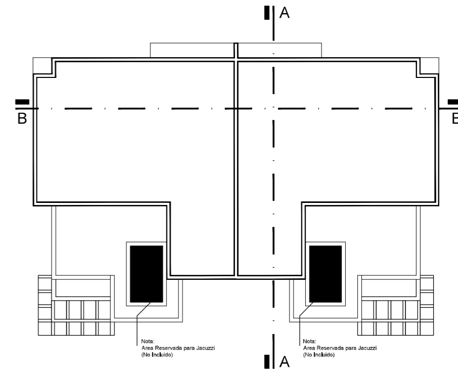
Planta de Techo Vivienda Duplex - Modelo A ESC 1:75
