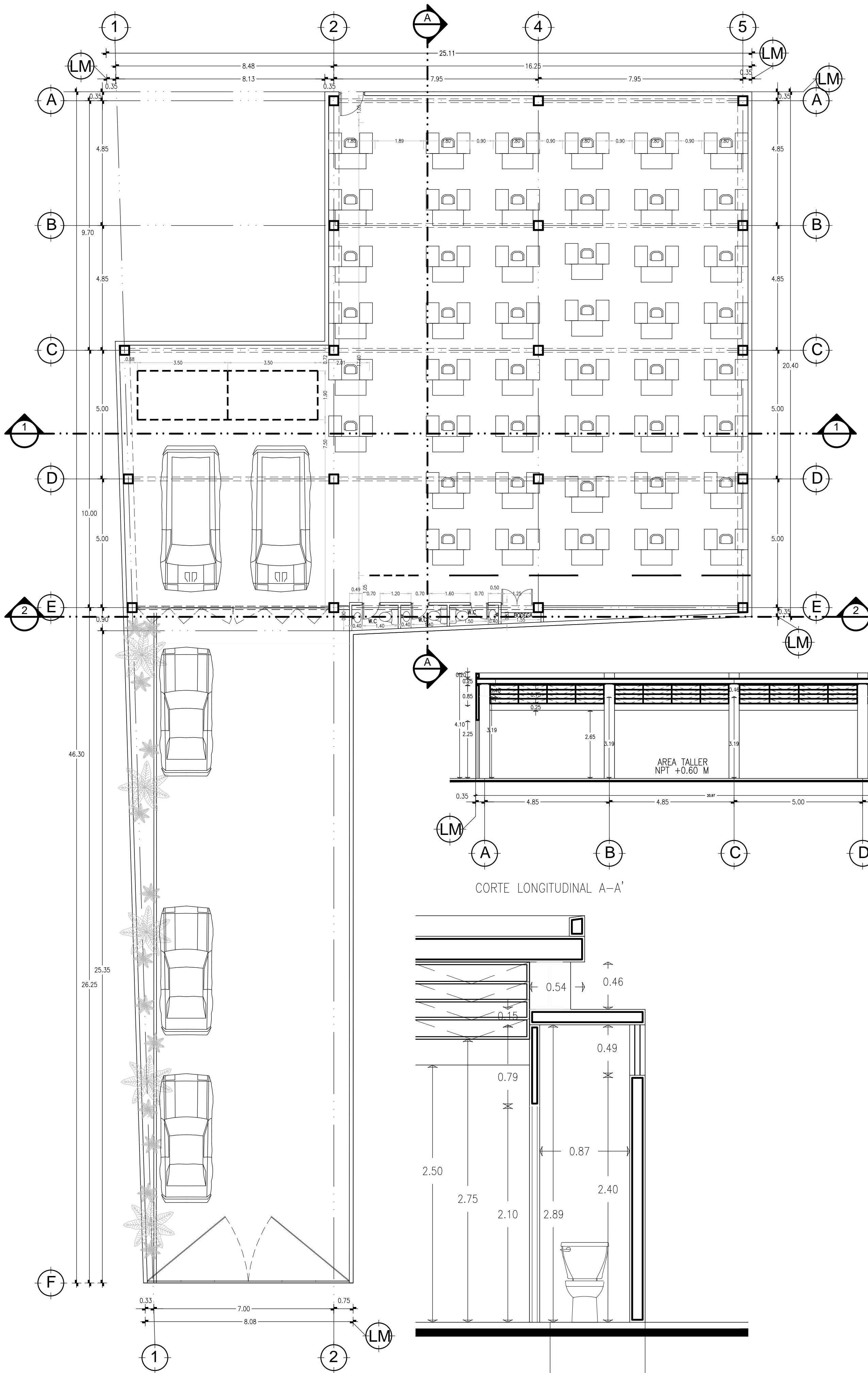
PLANTA ARQUITECTONICA TALLER TEKIT
