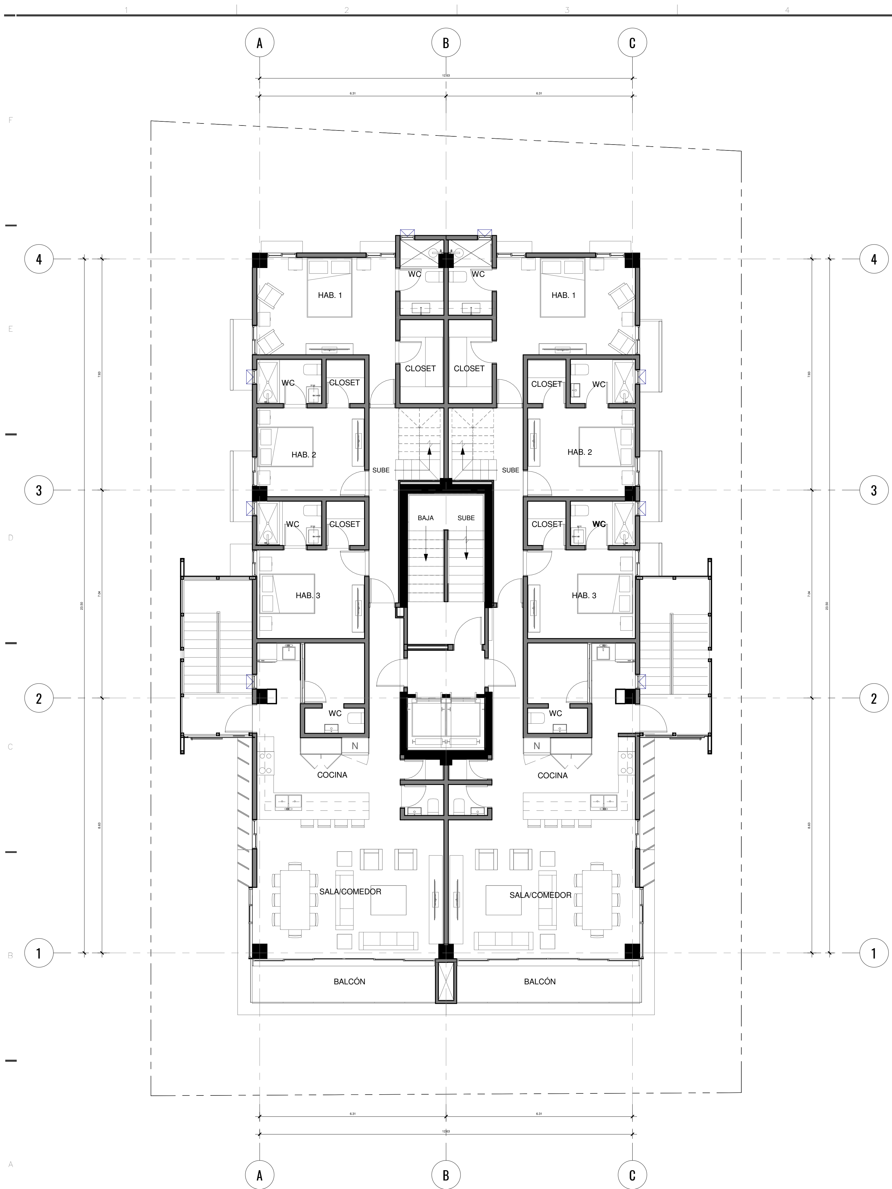
1 Nivel 10 - Penthouse N1 1:75
