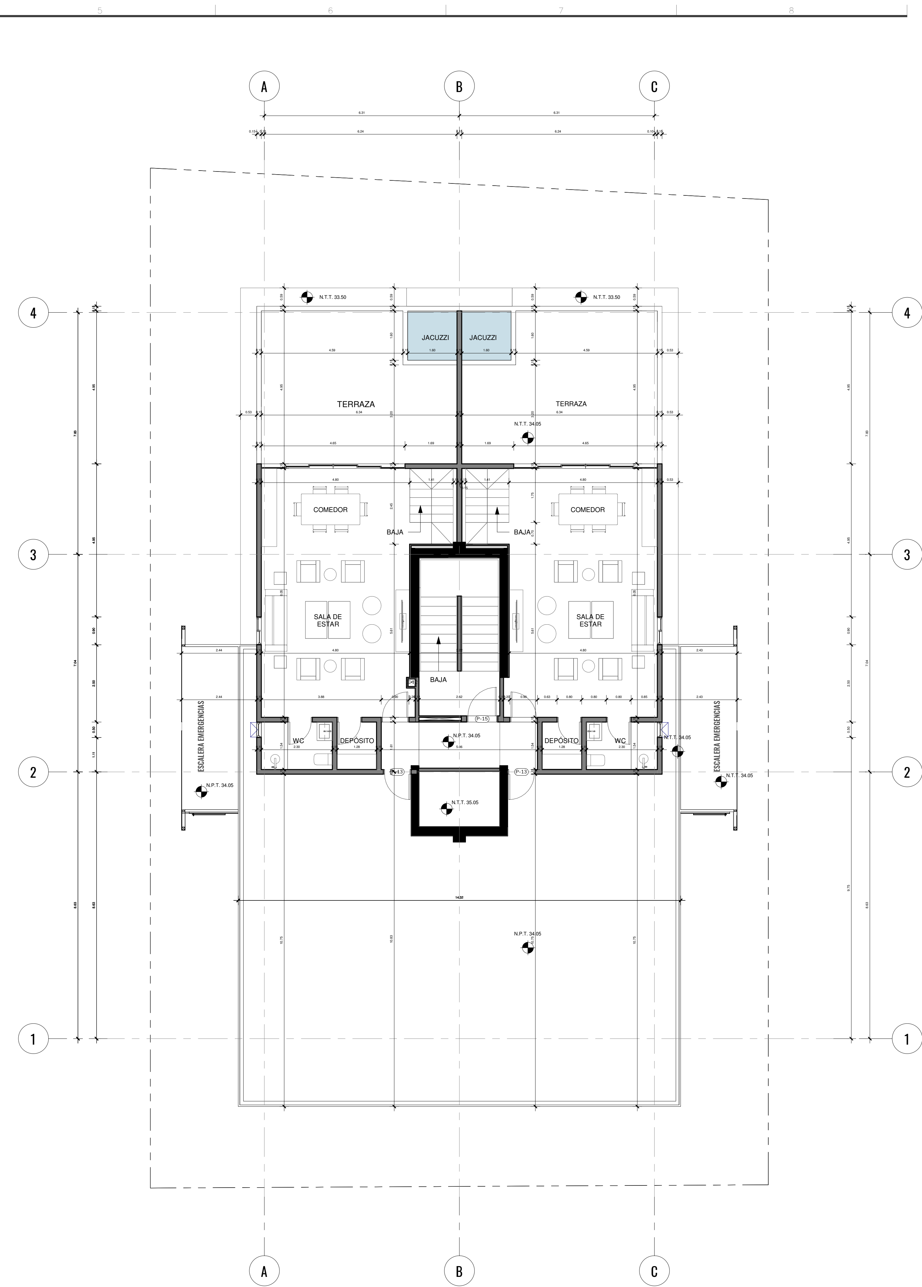
2 Nivel Azotea PH - Dimensionada 1:75
