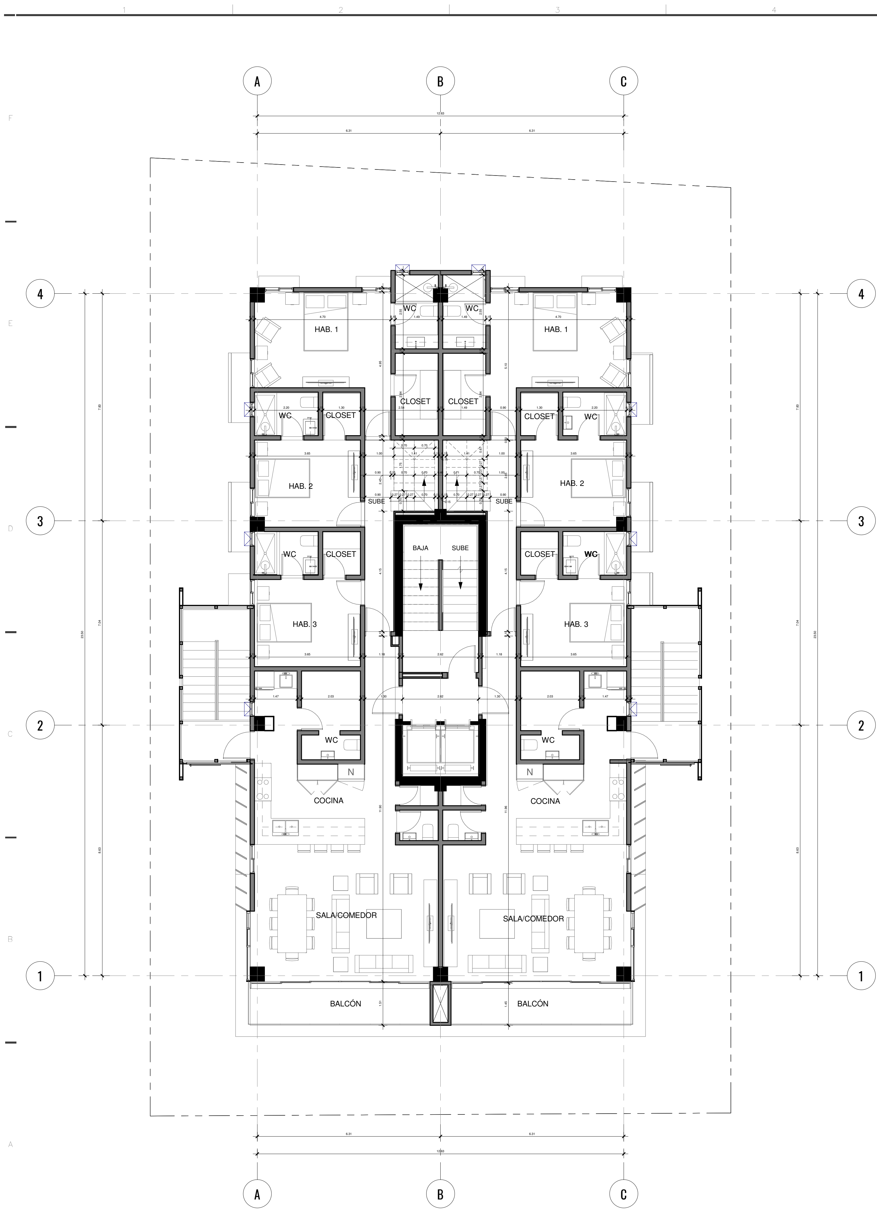
1 Nivel Penthouse - Dimensionada 1:75
