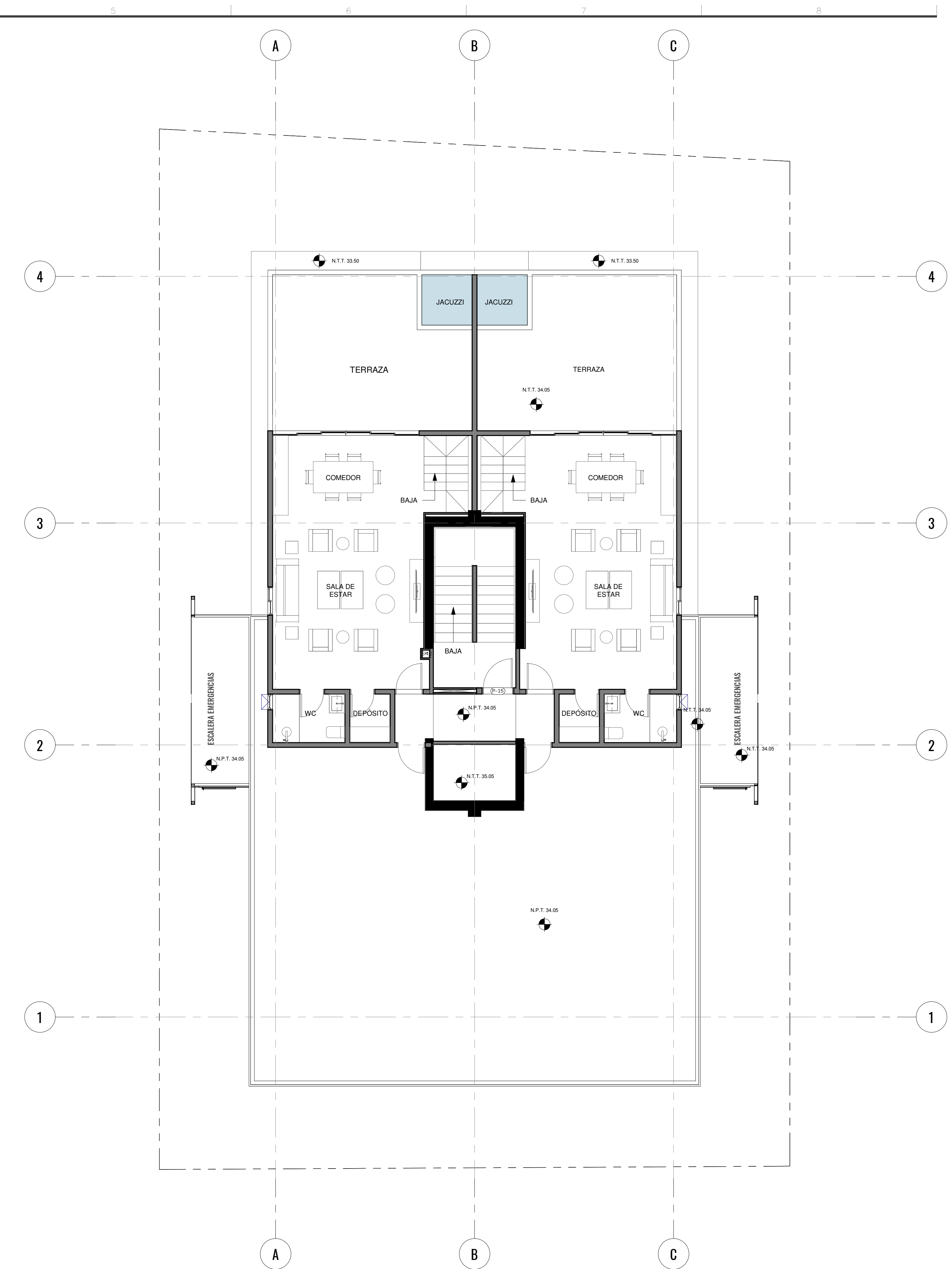
2 Nivel Azotea - PH 1:75
