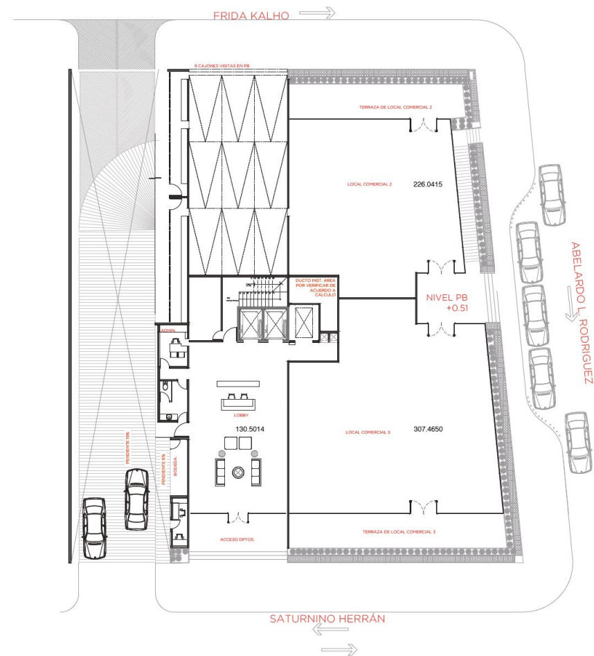
PLANTA BAJA
