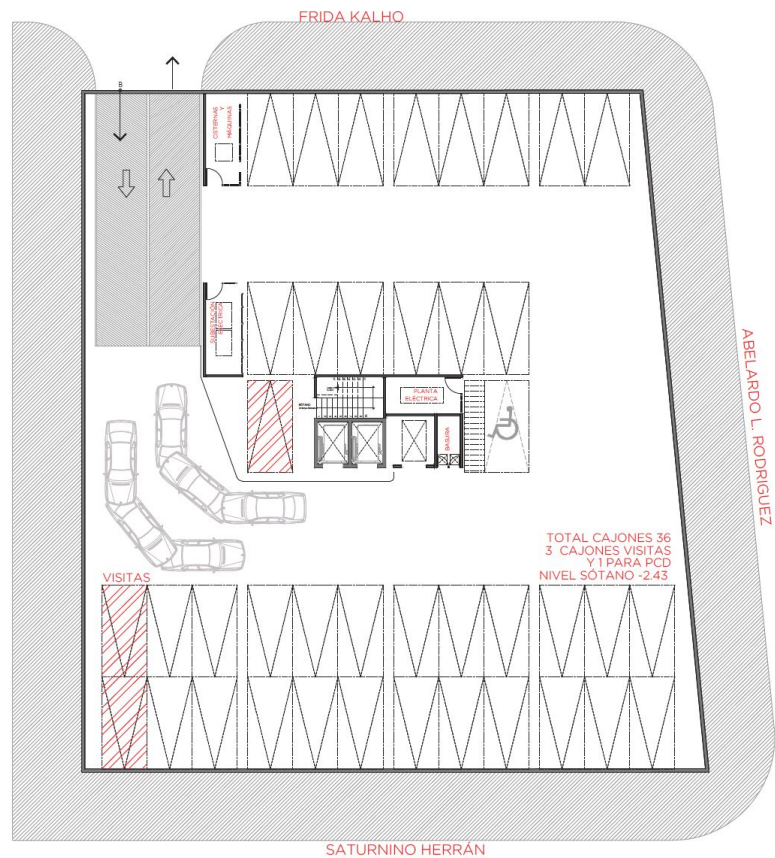
PLANTA SÓTANO
