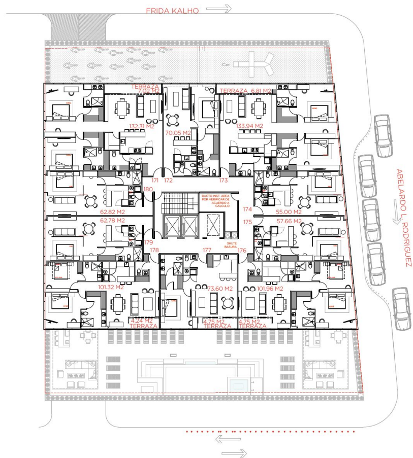
PLANTA TIPO 3 N17-N20
