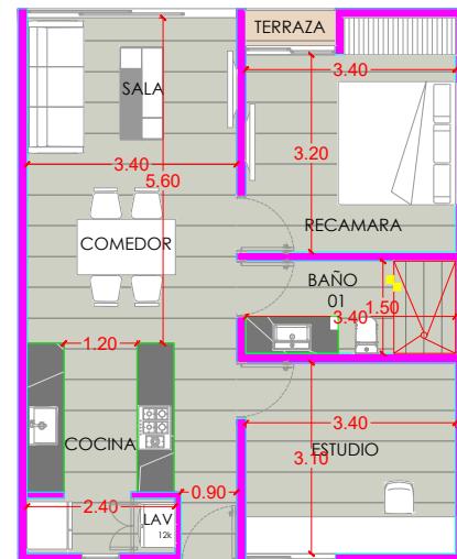
TIPO B
