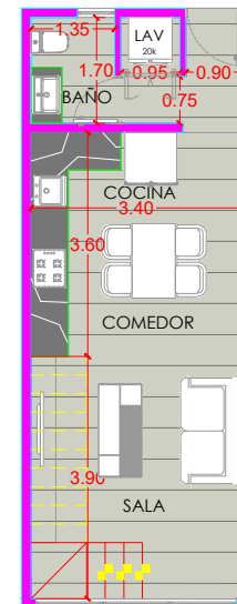
DUPLEX A
