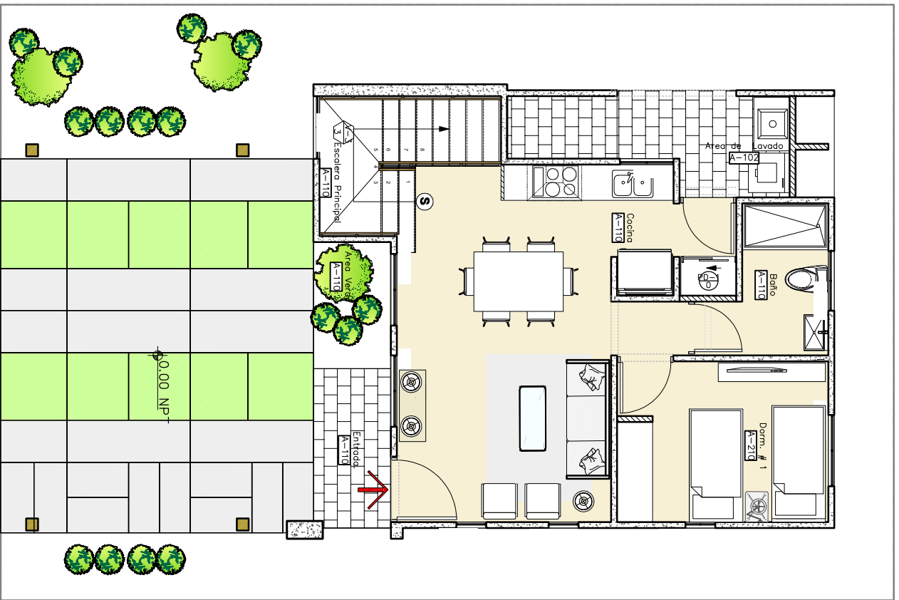
A P-1 PLANO AMUEBLADO 1ER NIVEL (TIPO C) Scale: 1:50
