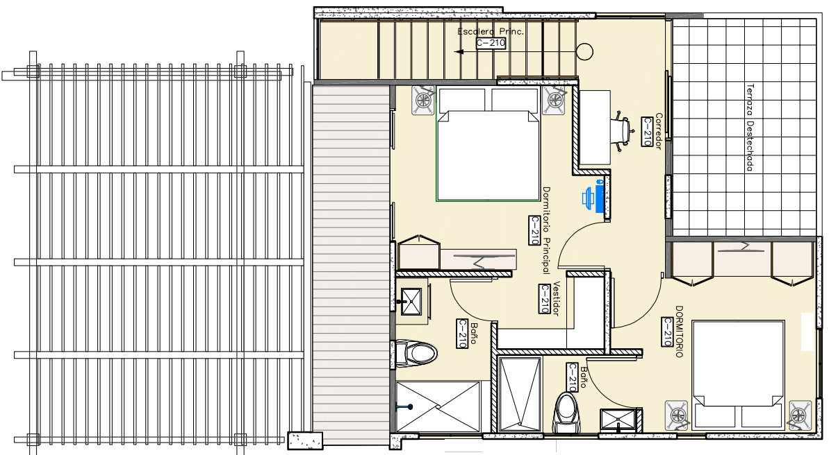
A P-1 PLANO AMUEBLADO 2DO NIVEL (TIPO C) Scale: 1:50
