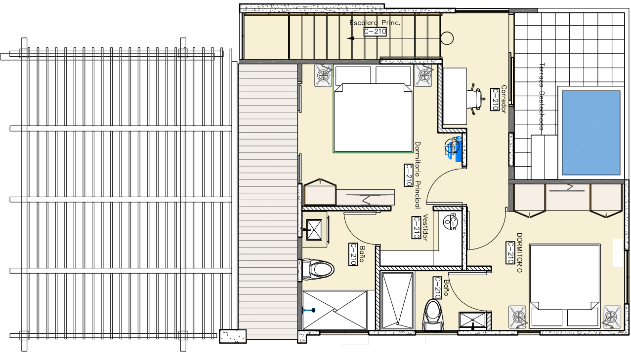
A P-1 PLANO AMUEBLADO 2DO NIVEL (TIPO C) Scale: 1:50
