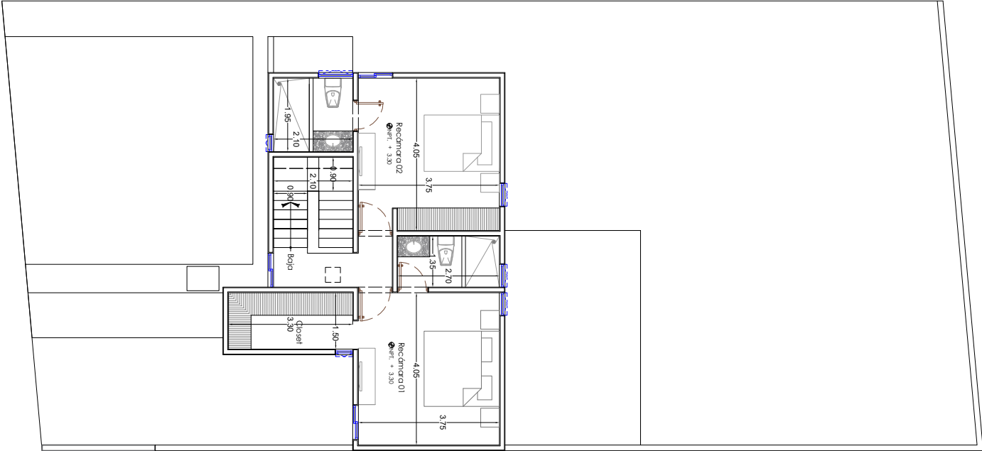
PLANTA ALTA
