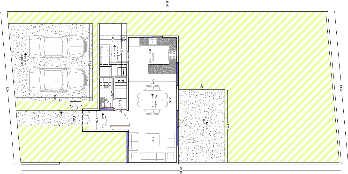
PLANTA BAJA
