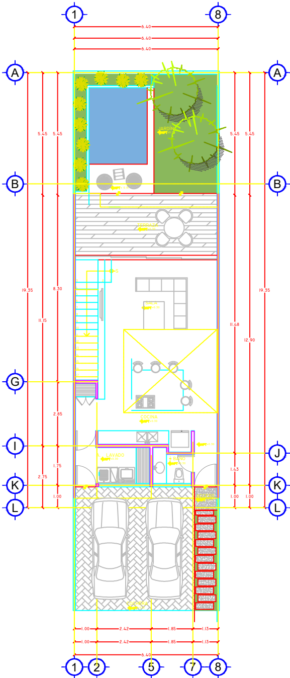
LOFT I PLANTA BAJA
