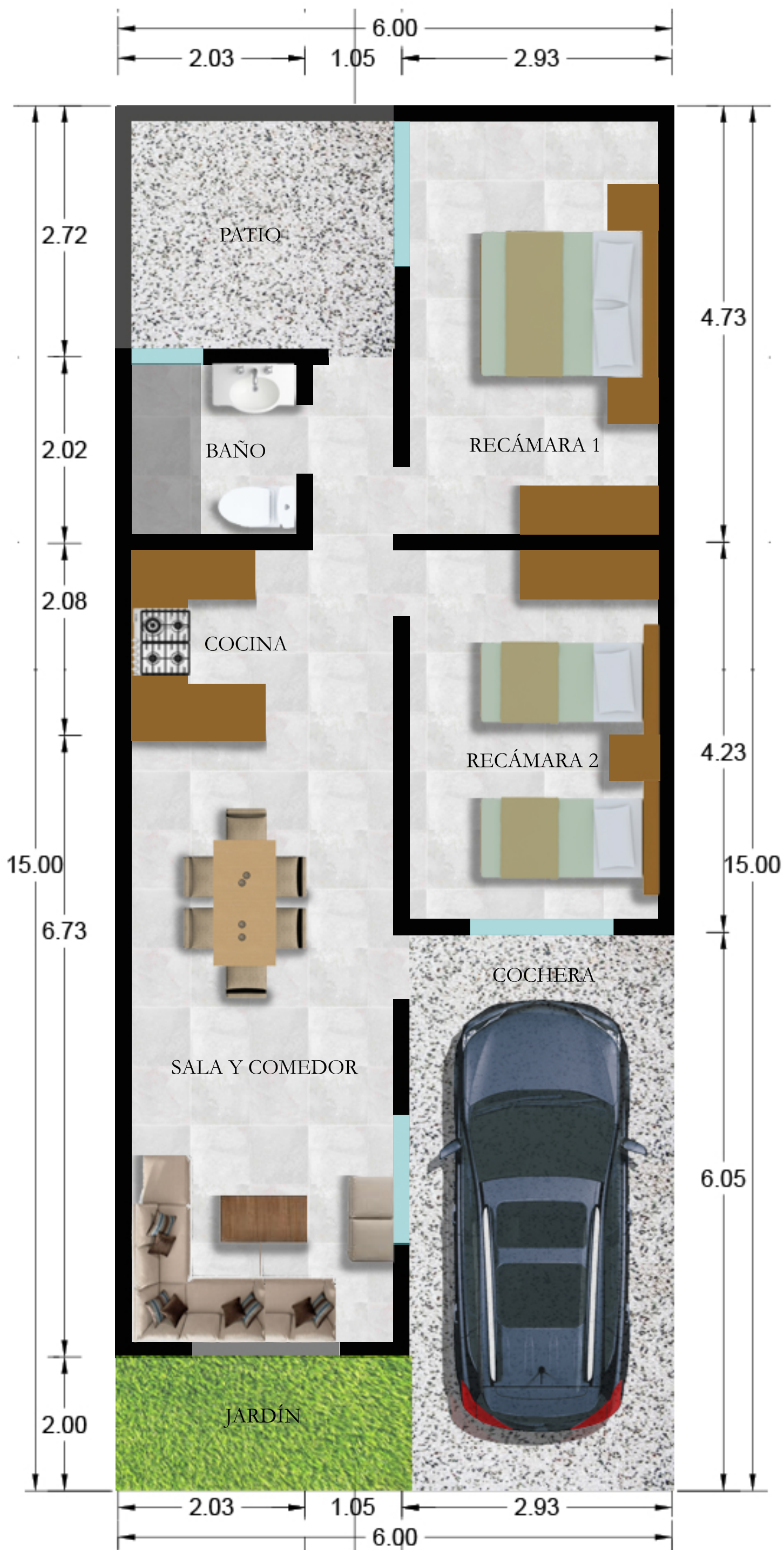
PLANTA GENERAL DE VIVENDA
