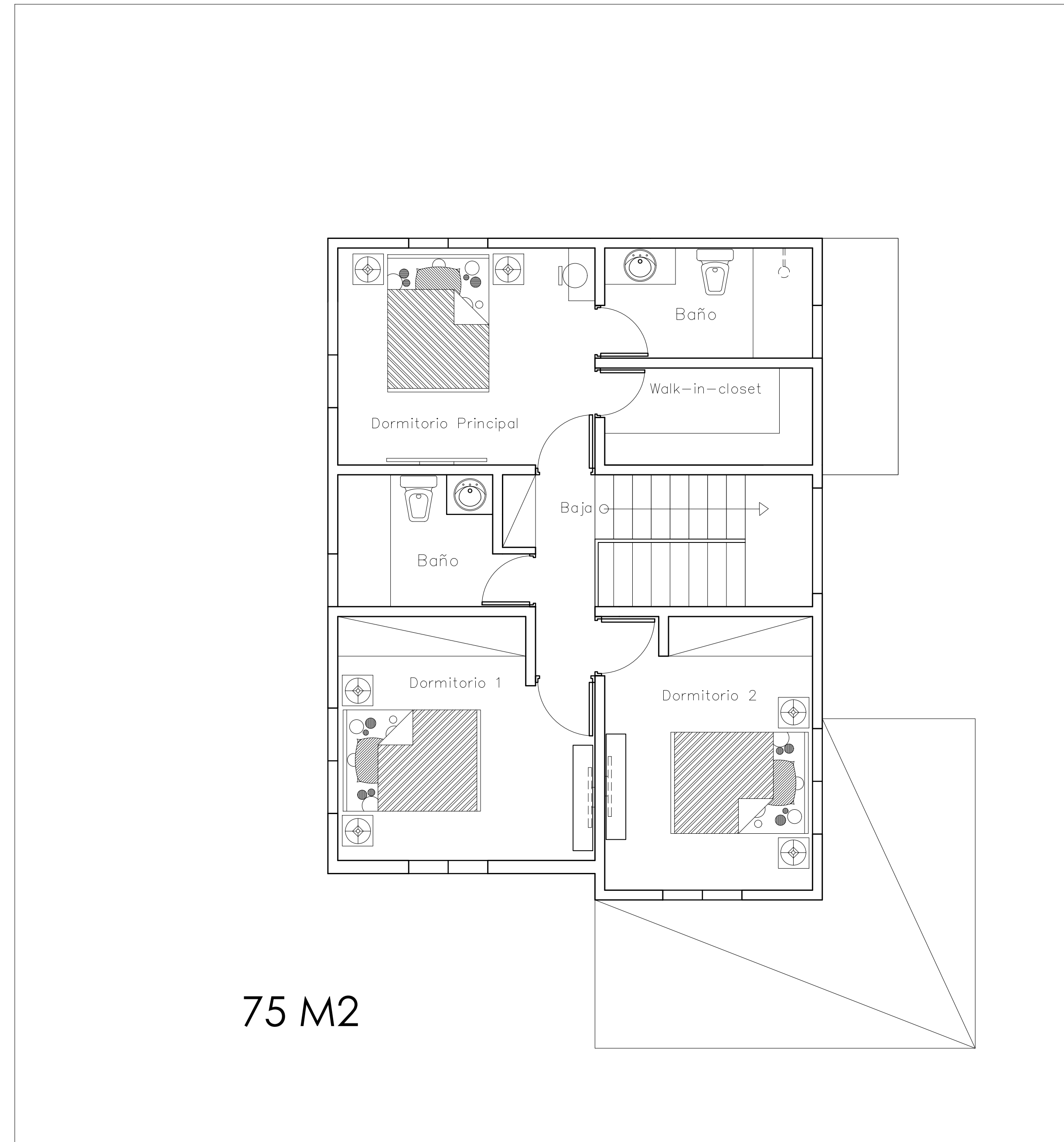
PLANTA ARQUITECTONICA AMUEBLADA DE CONJUNTO Nivel 2
