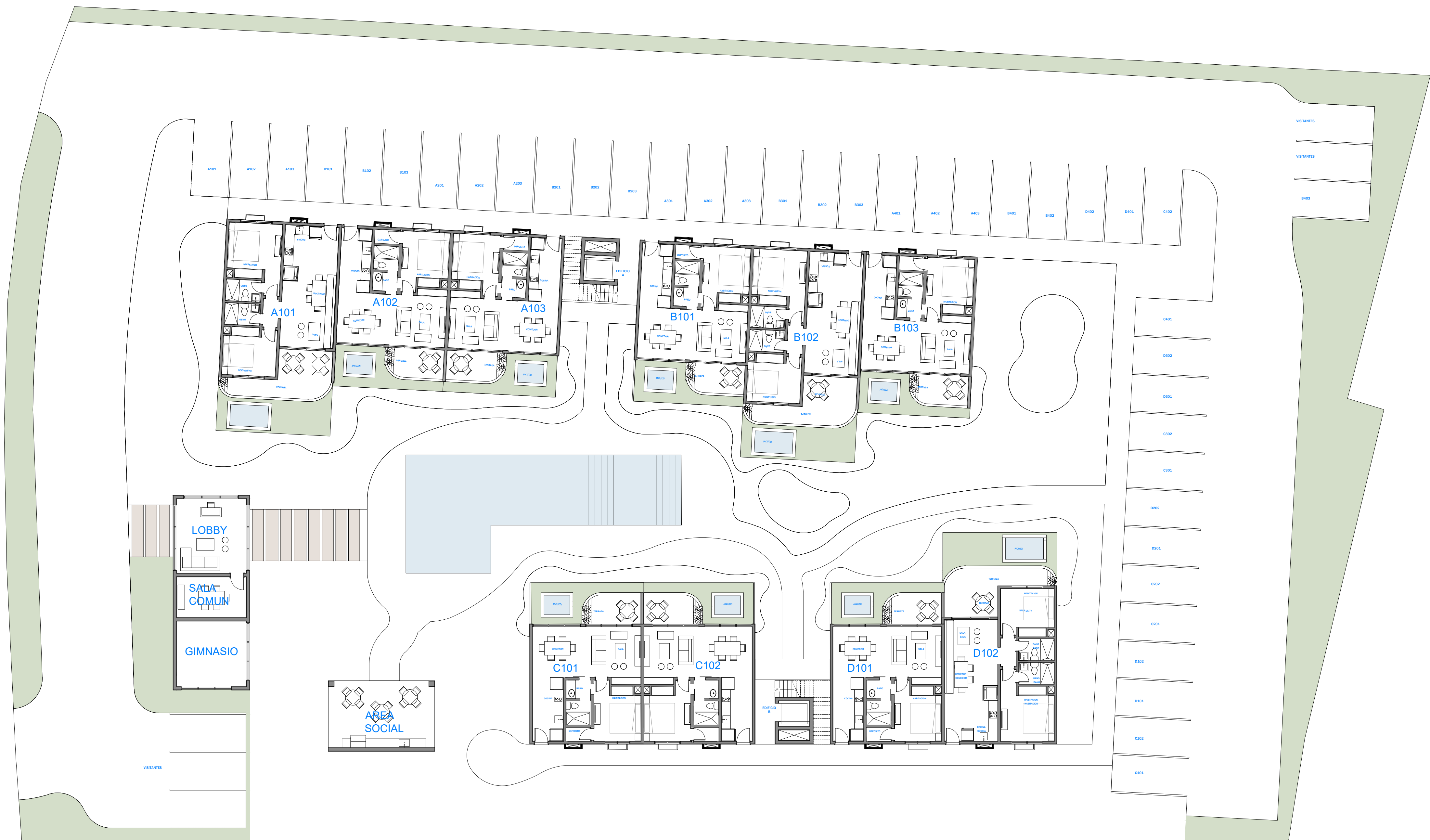
PLANTA DE CONJUNTO NIVEL 1 ESC: 1/200
