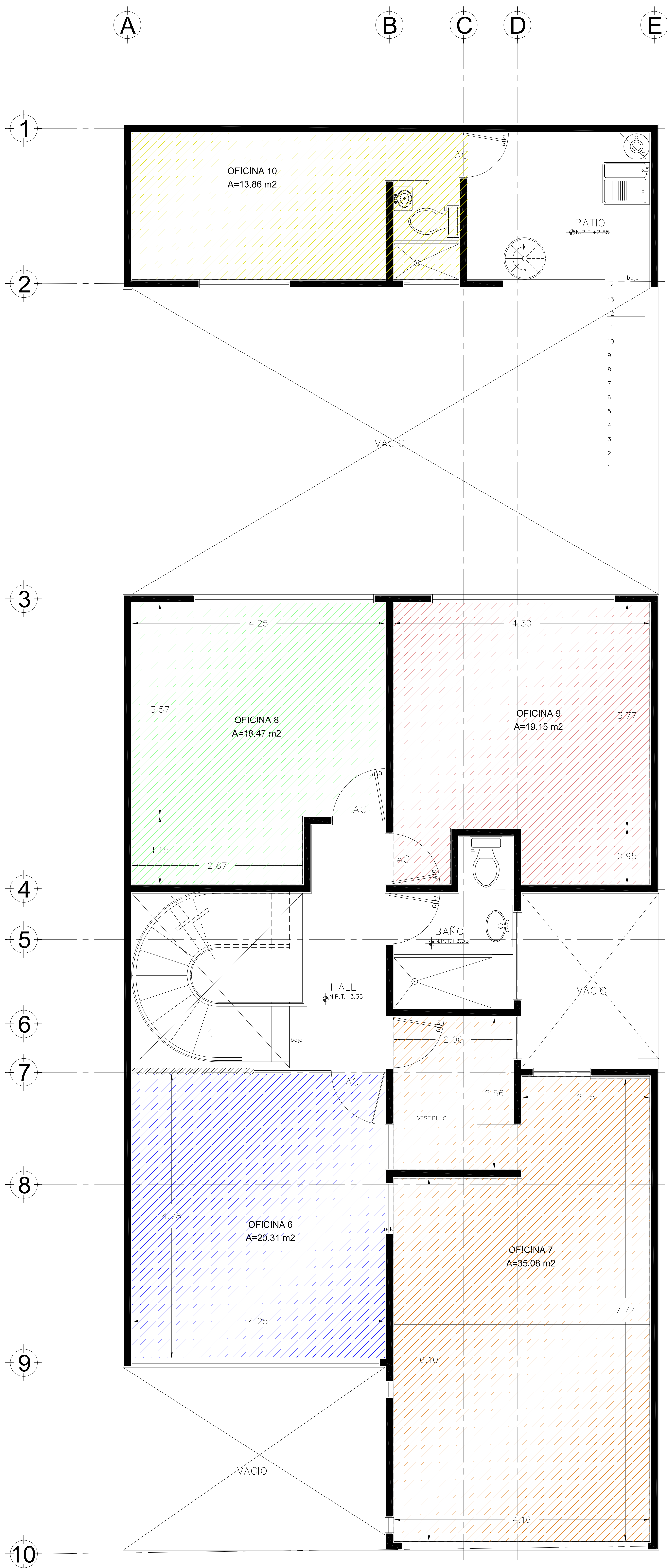
PLANTA ALTA
