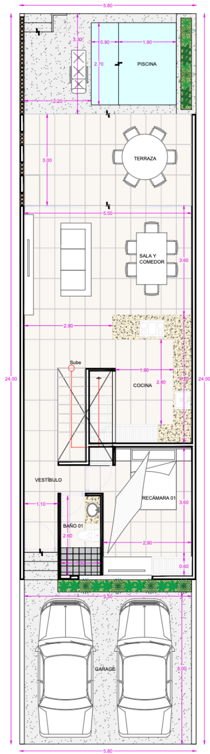
PLANTA BAJA
