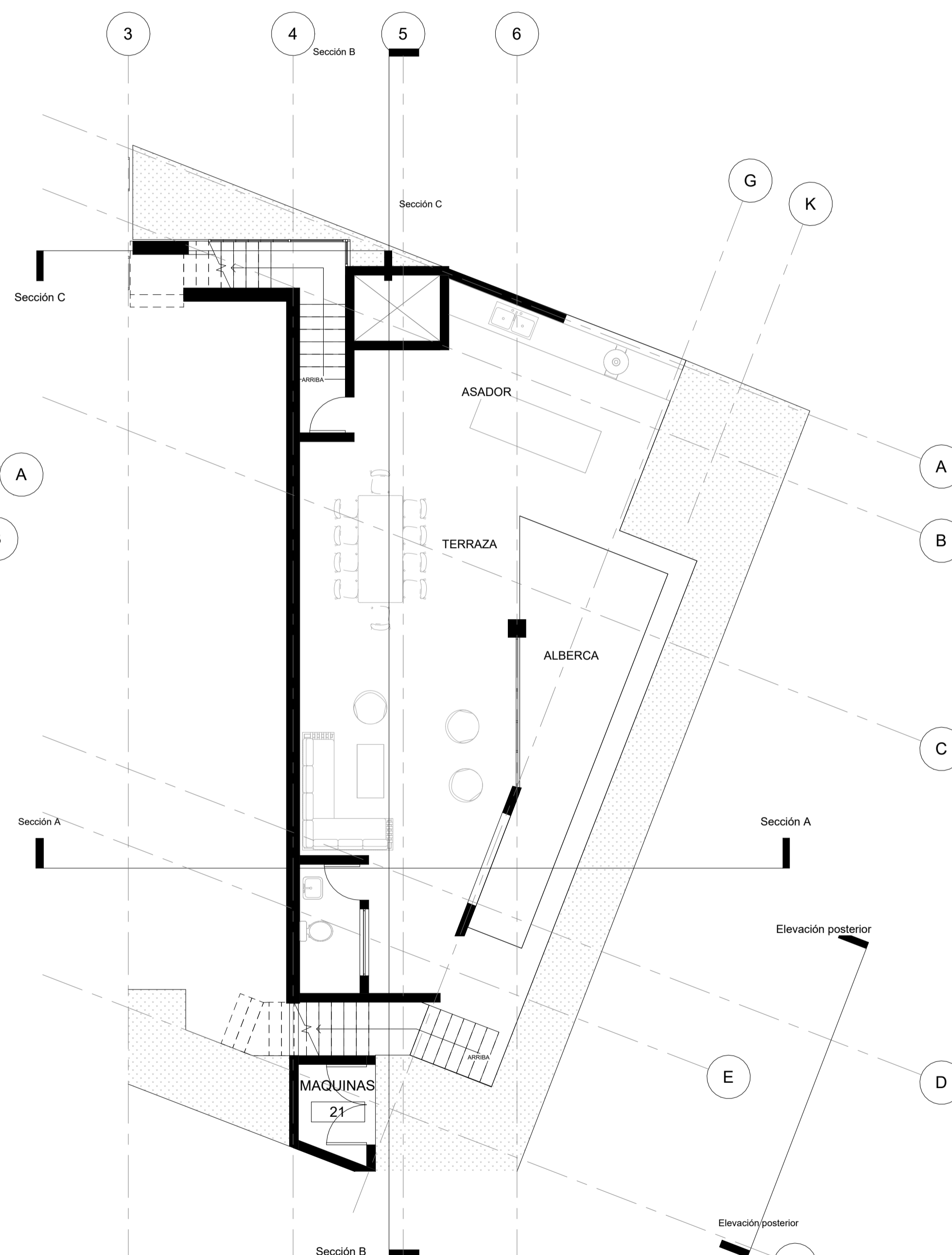
2 AREA SOCIAL 2 1 : 75
