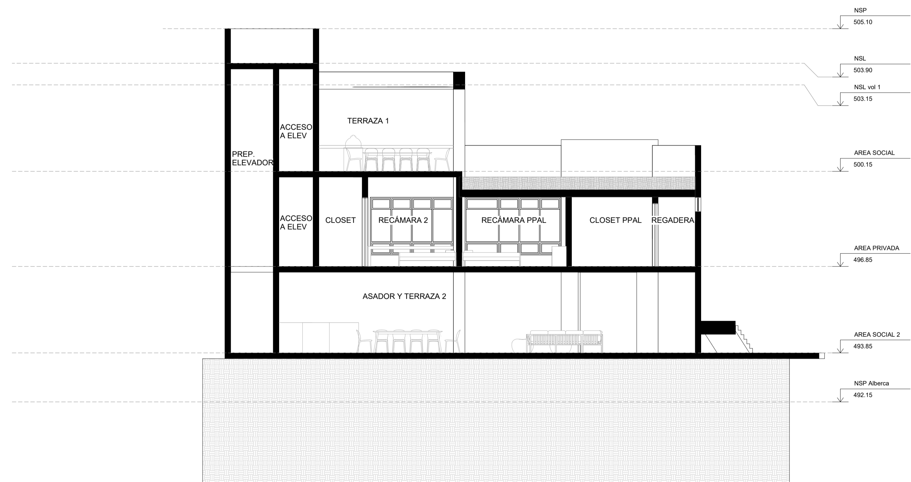
2 Sección B 1 : 75
