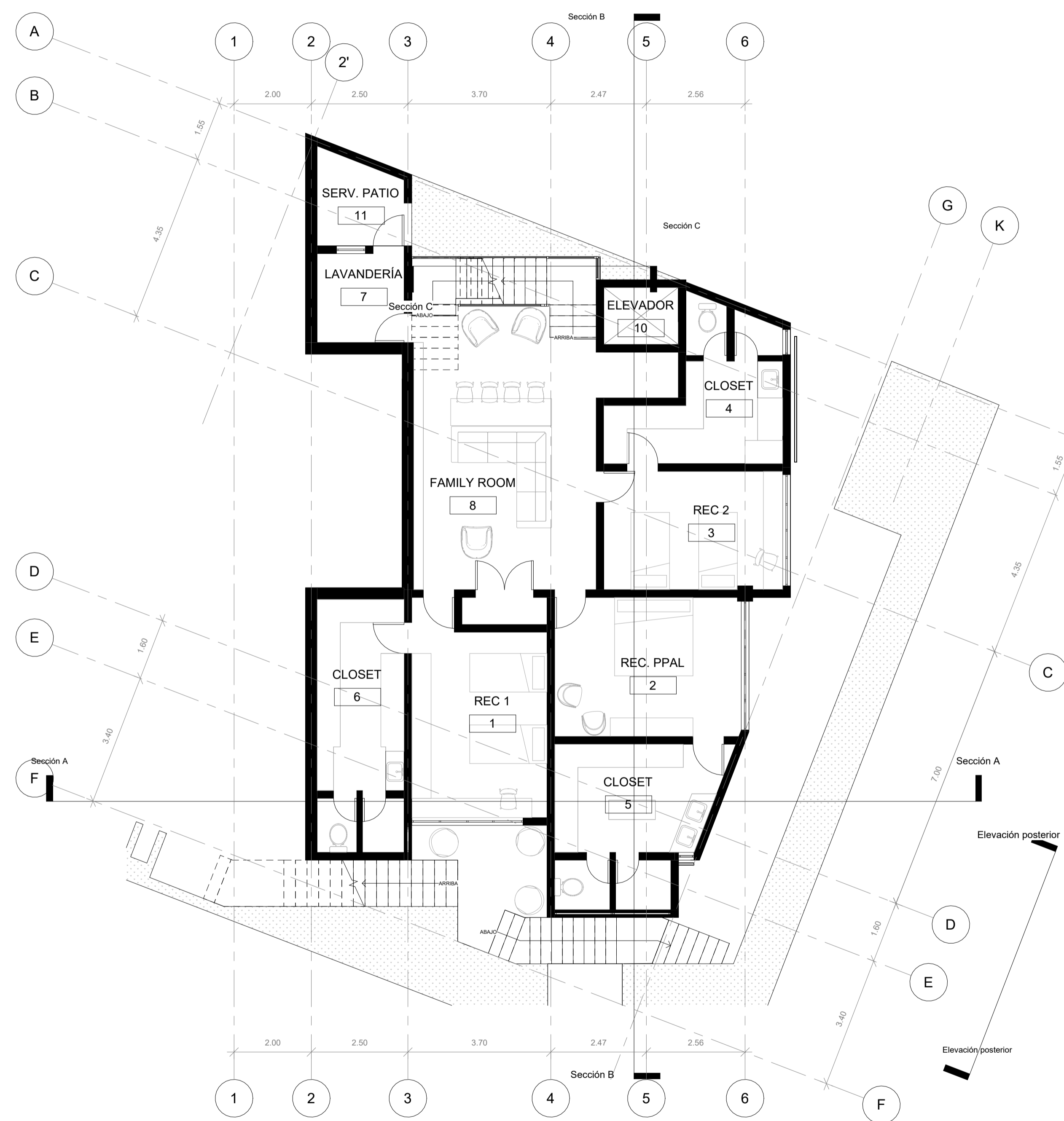
1 AREA PRIVADA 1 : 75
