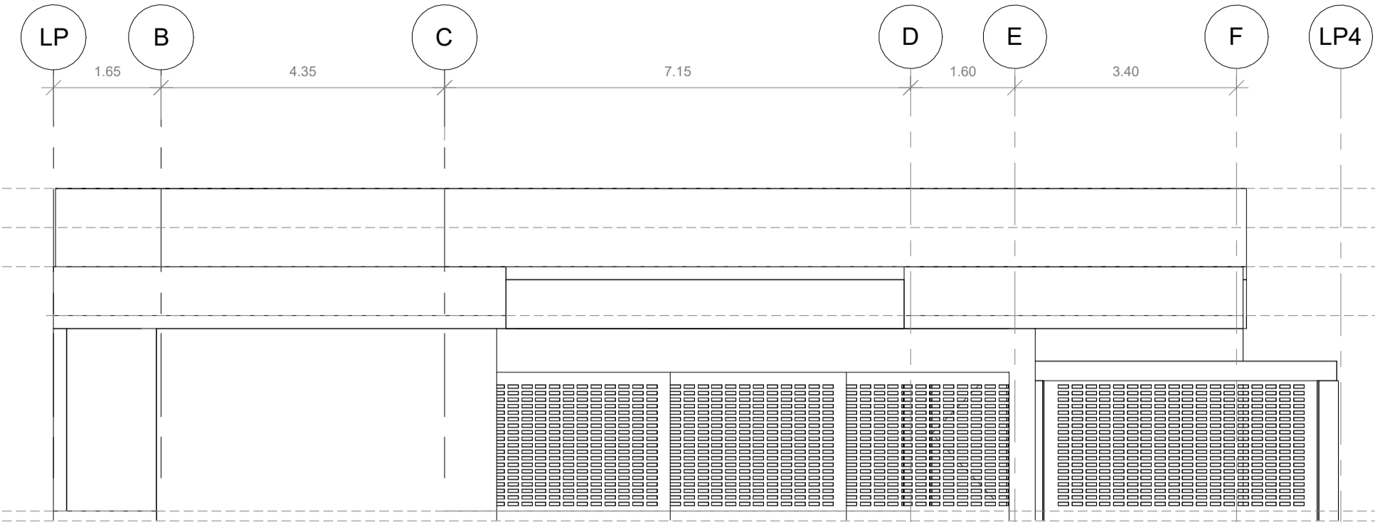
1 Elevación frontal 1:75
