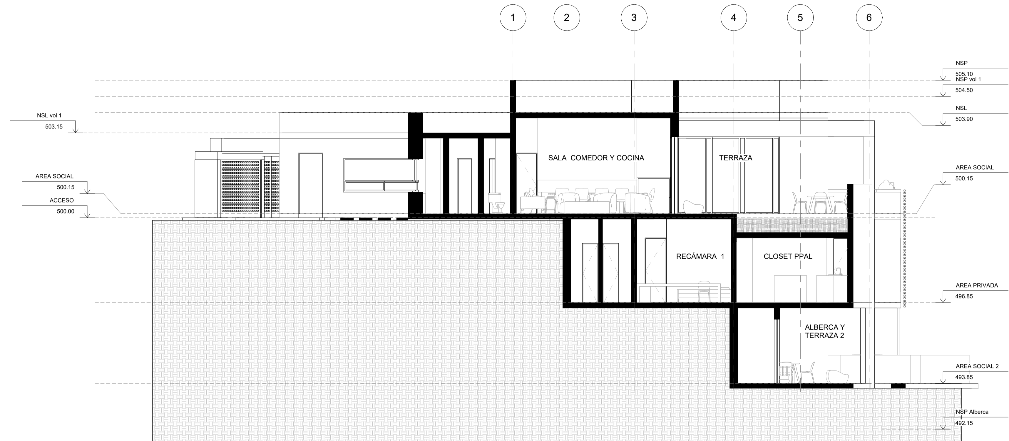
1 Sección A 1 : 75
