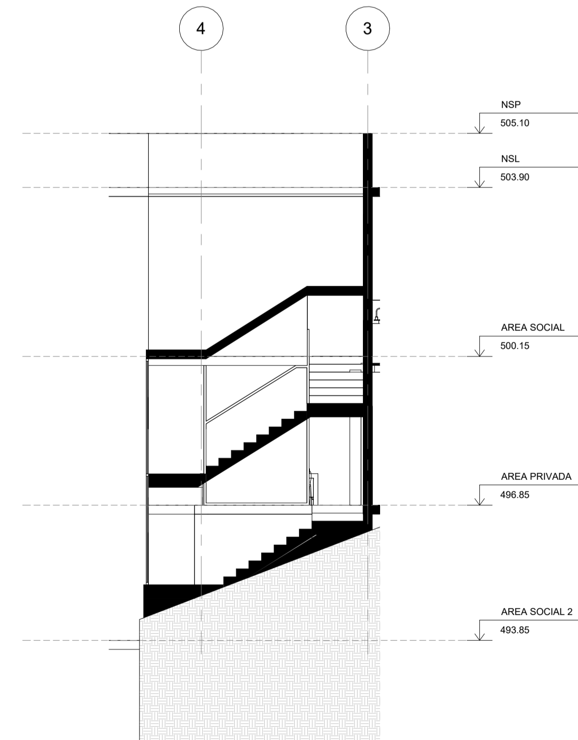
3 Sección C 1 : 75
