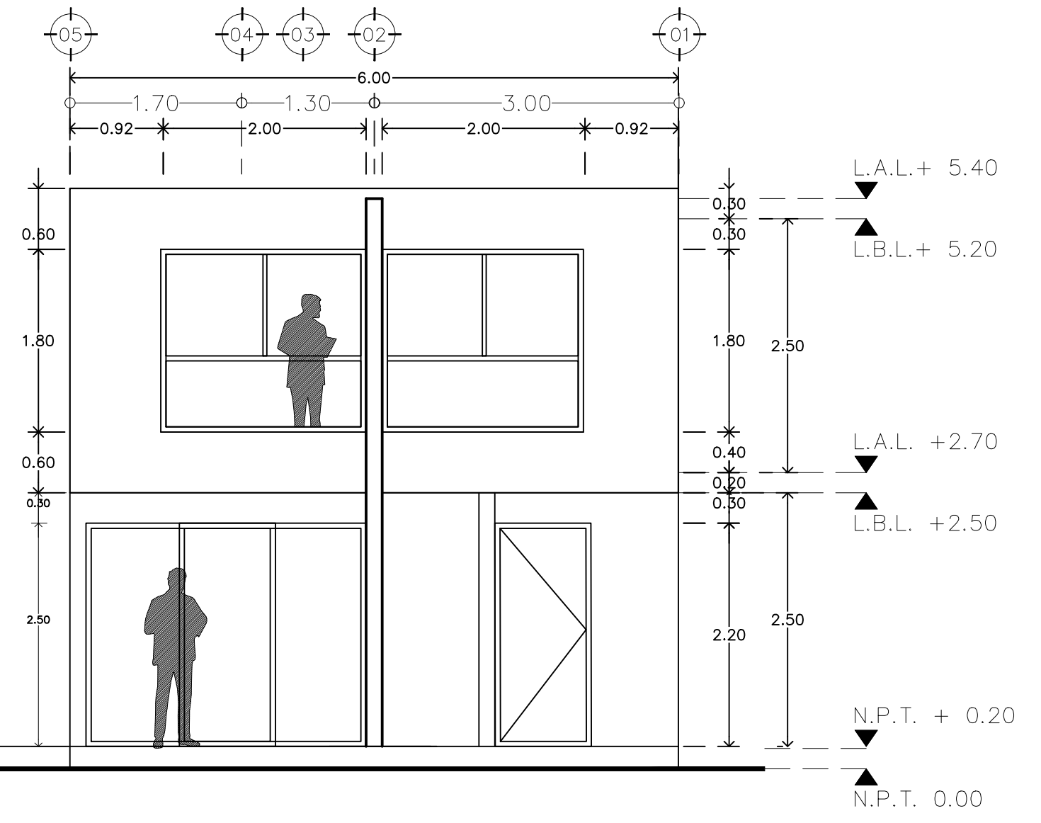
ALZADO POSTERIOR
