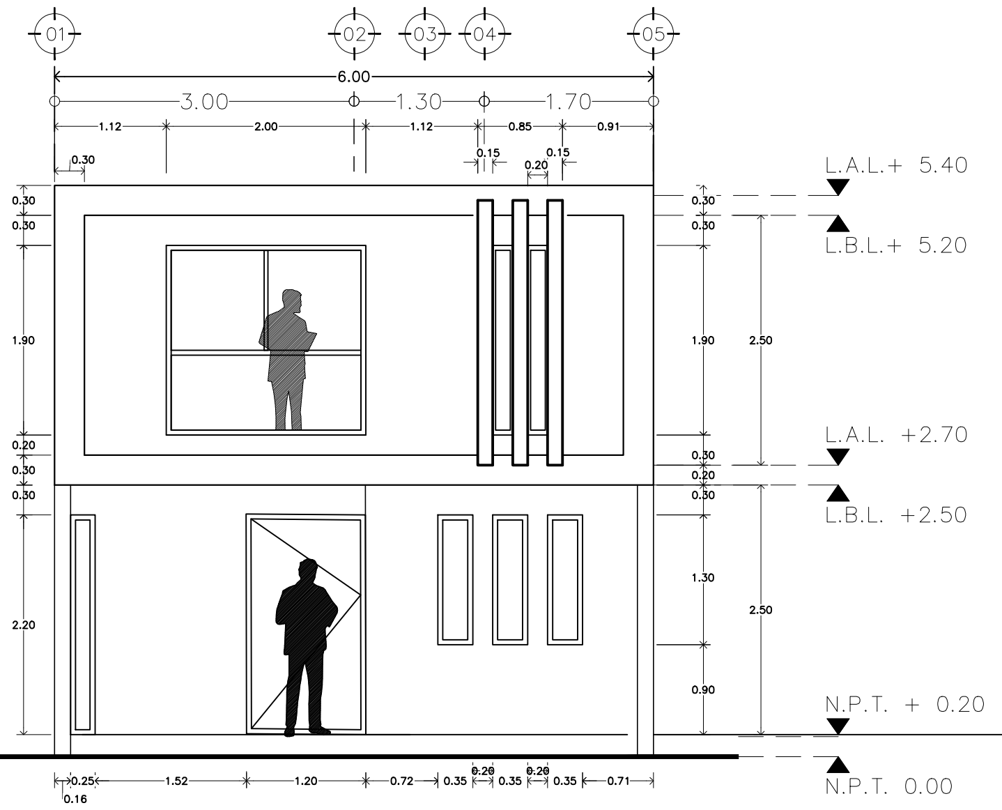
ALZADO FRONTAL
