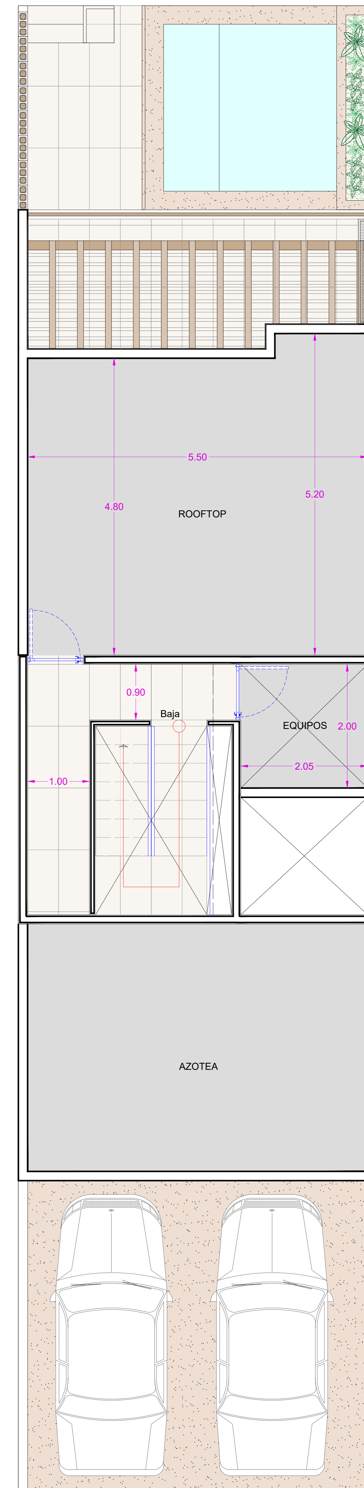
PLANTA SEGUNDO NIVEL
