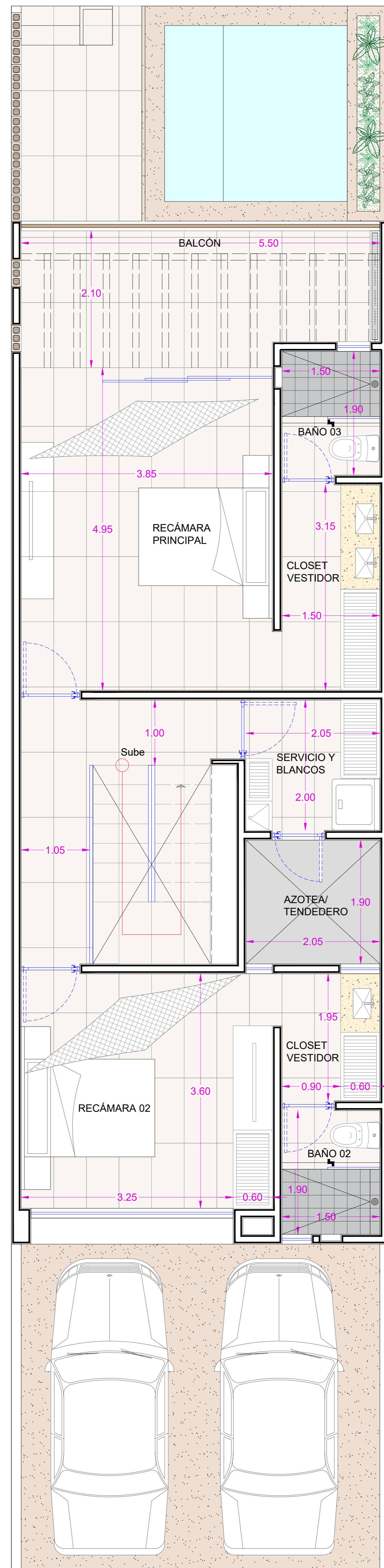
PLANTA PRIMER NIVEL
