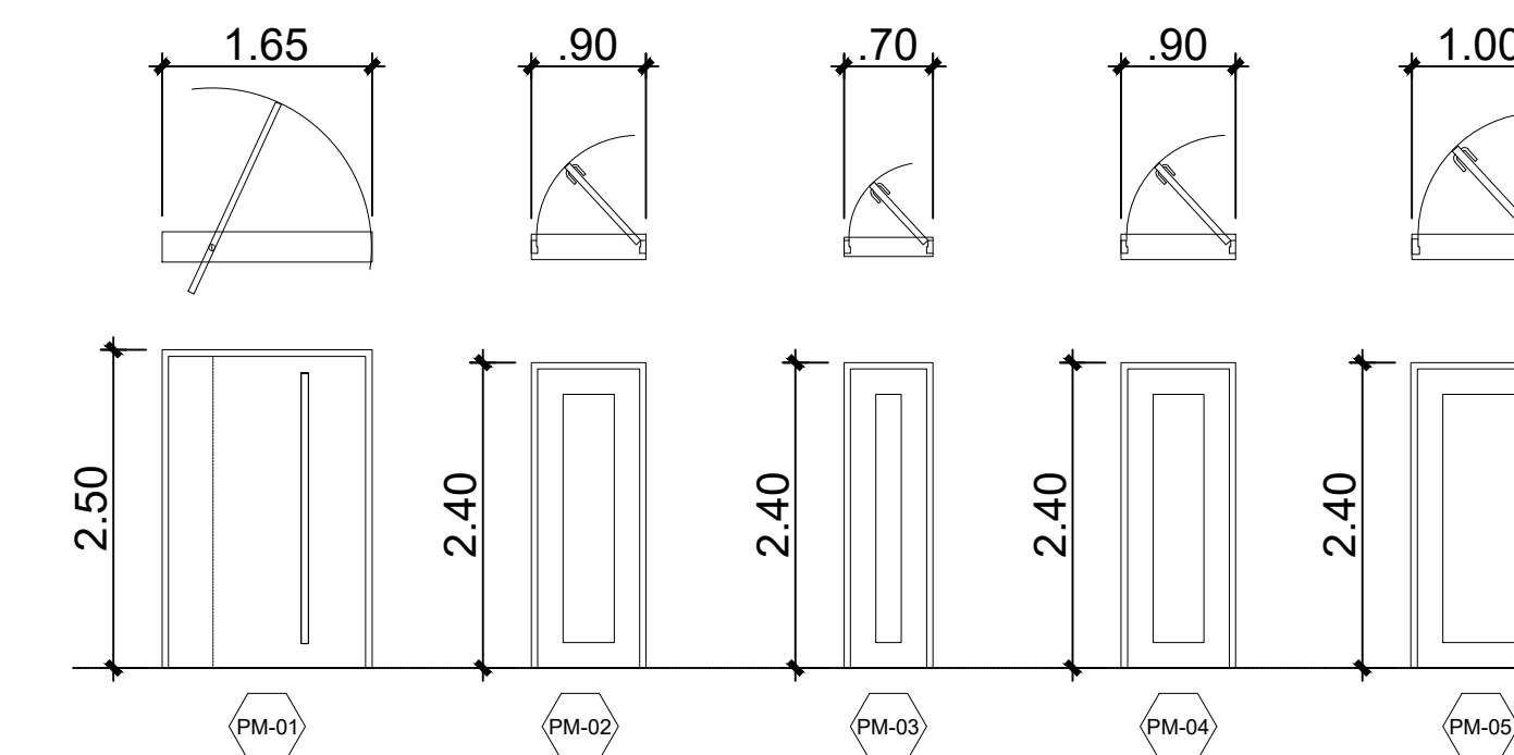
ELEVACIONES DE PUERTAS DE MADERA
