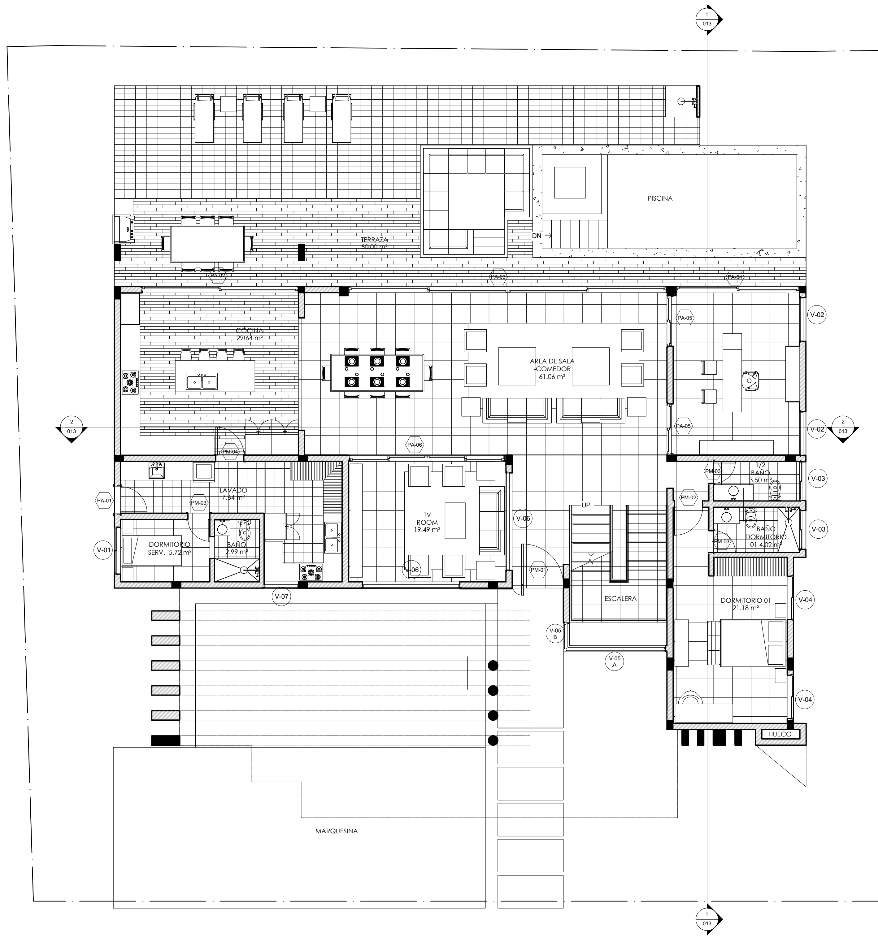
1 PLANO ARQUITECTONICO N01 1:75
