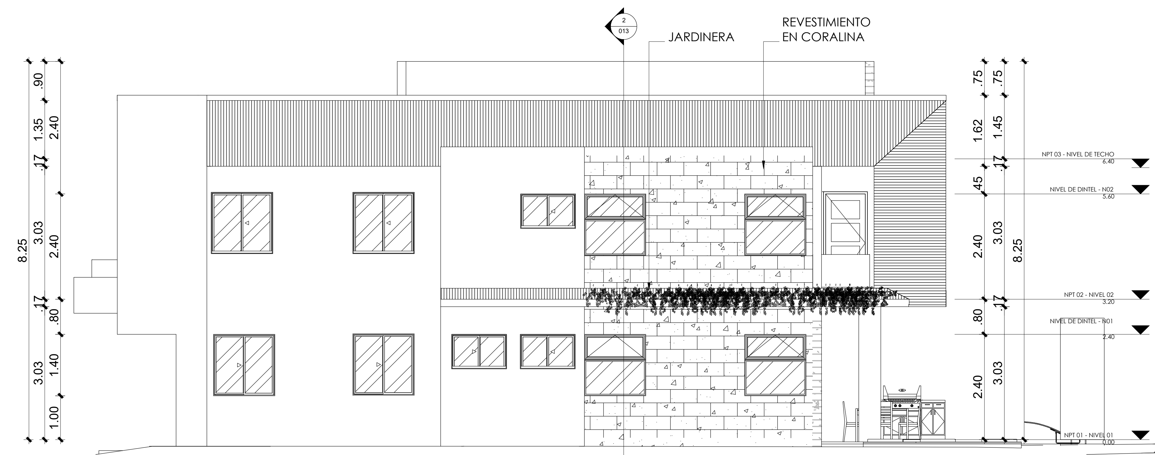
2 ELEVACION LAT. DERECHA 1 : 50
