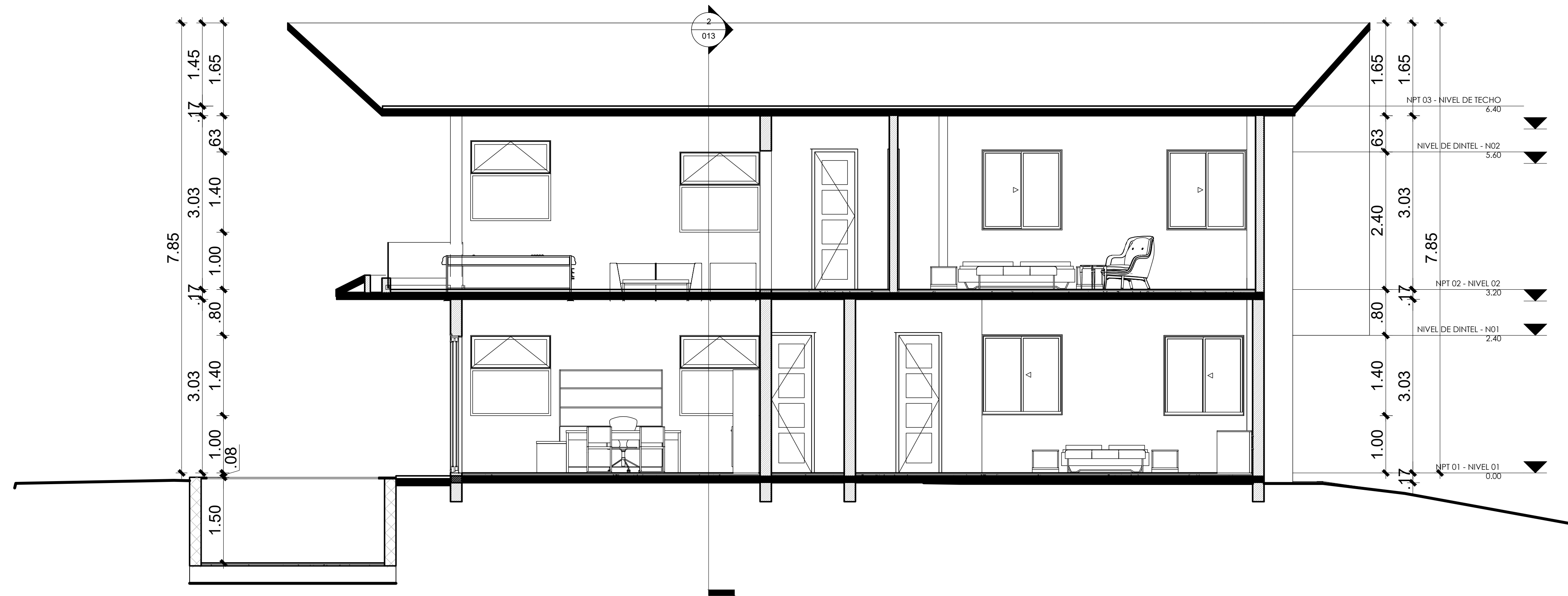
1 SECCION 01 1 : 50
