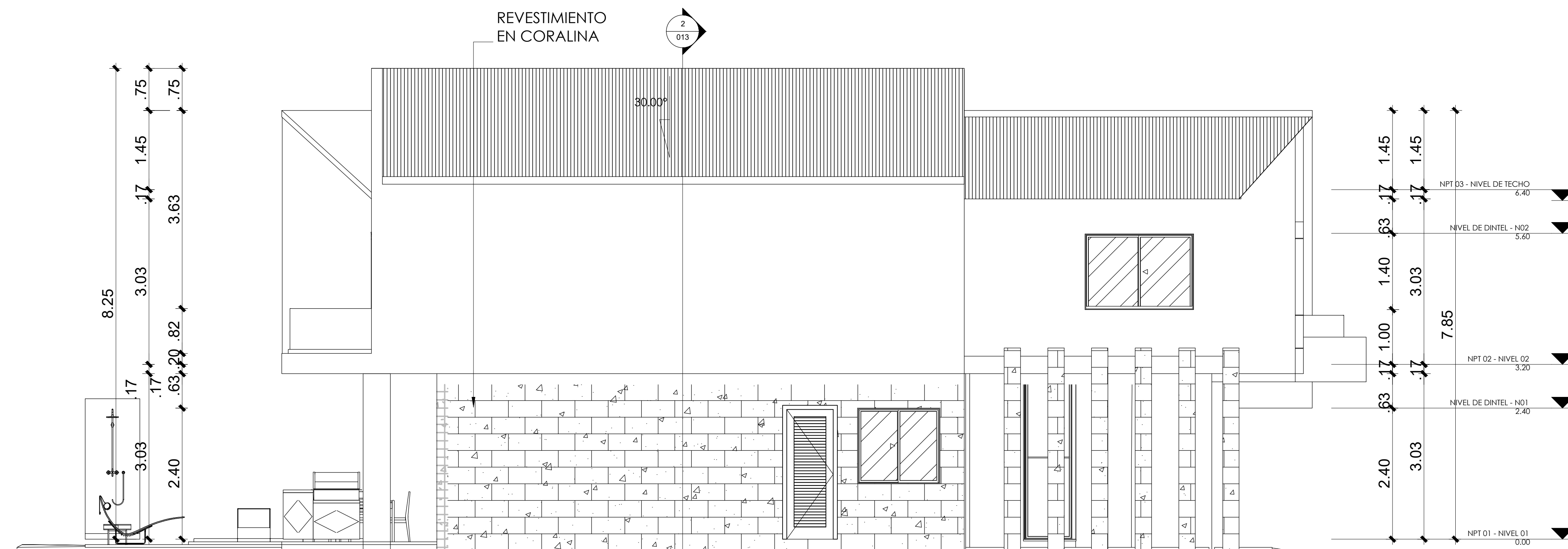
2 ELEVACION LAT. IZQUIERDA 1 : 50
