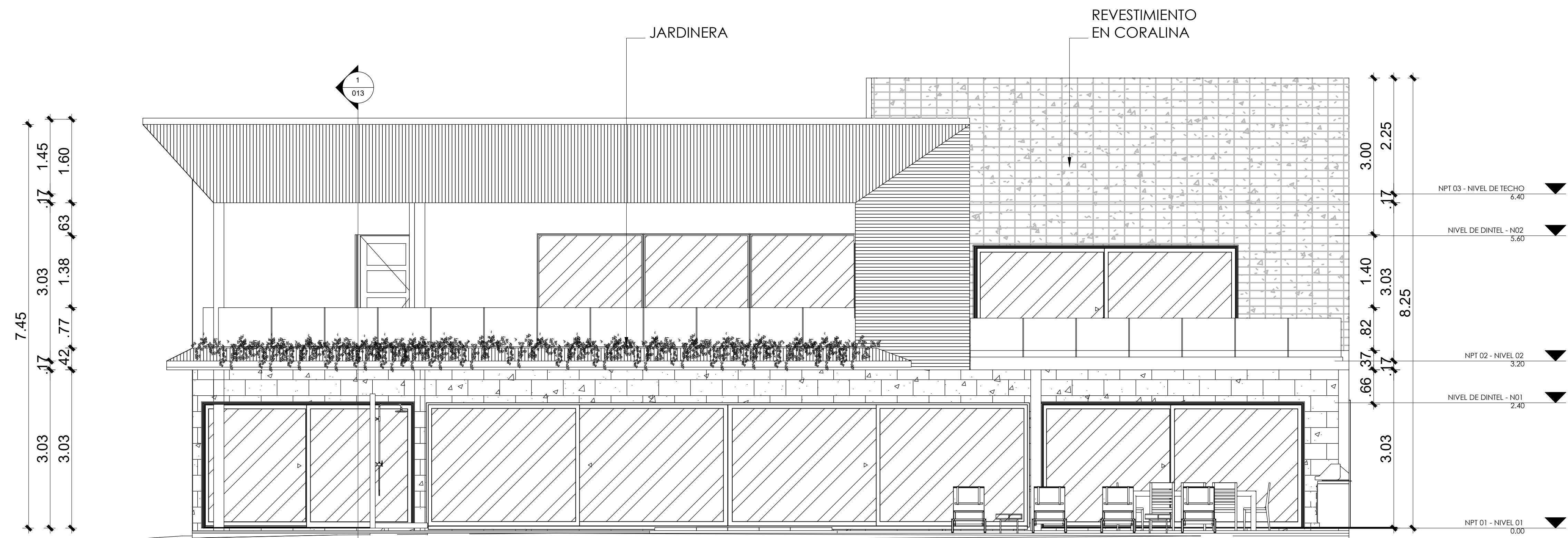
1 ELEVACION POSTERIOR 1 : 50
