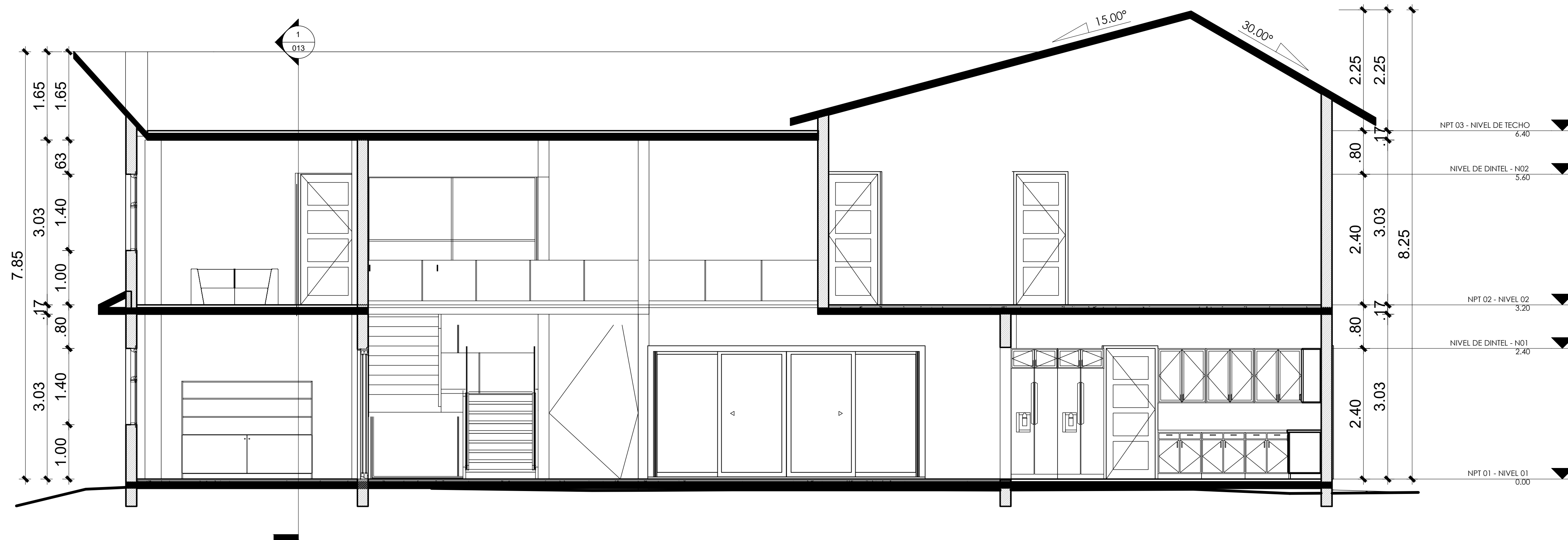
1 SECCION 02 1 : 50
