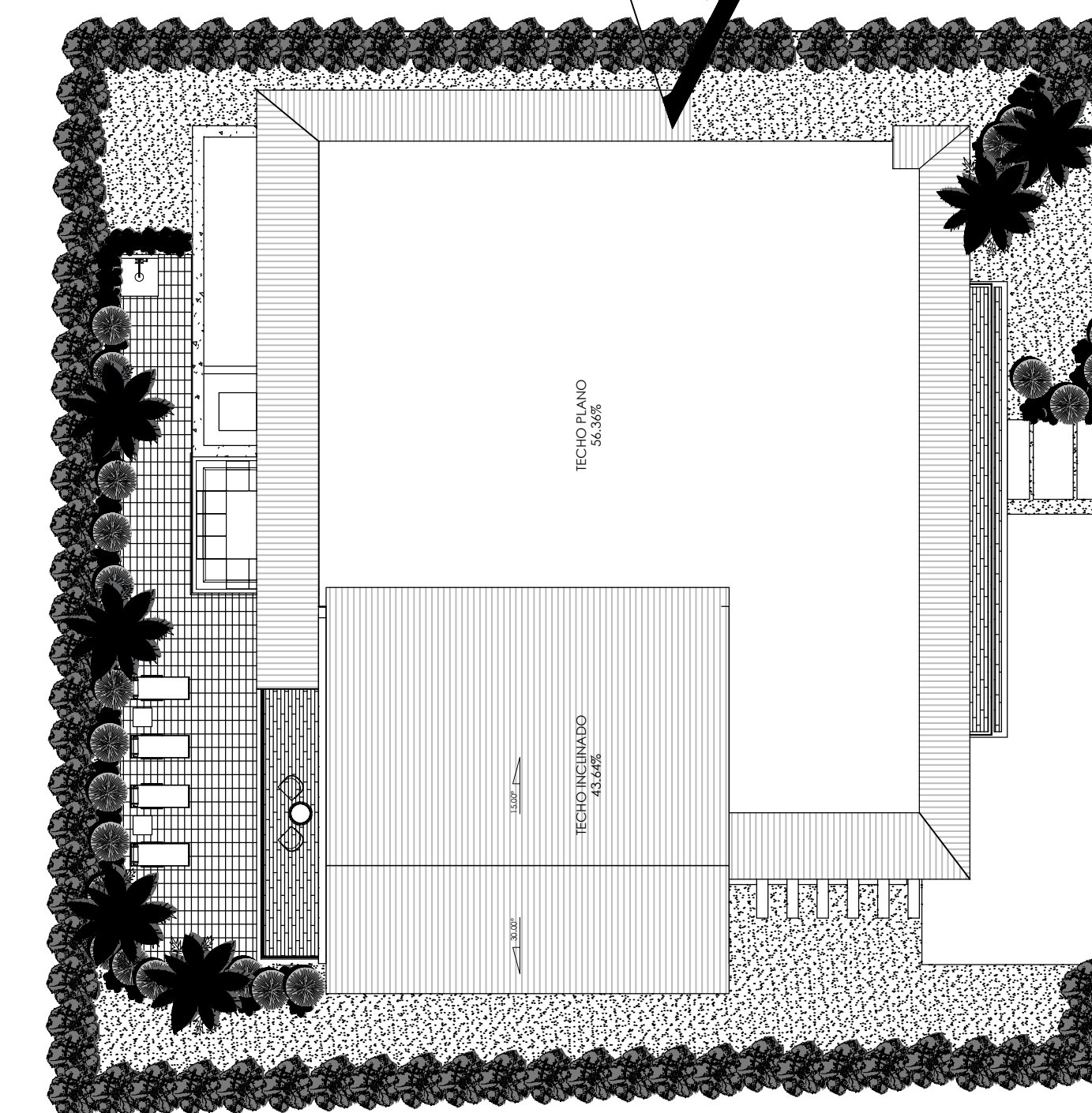
1 PLANO DE TECHO
