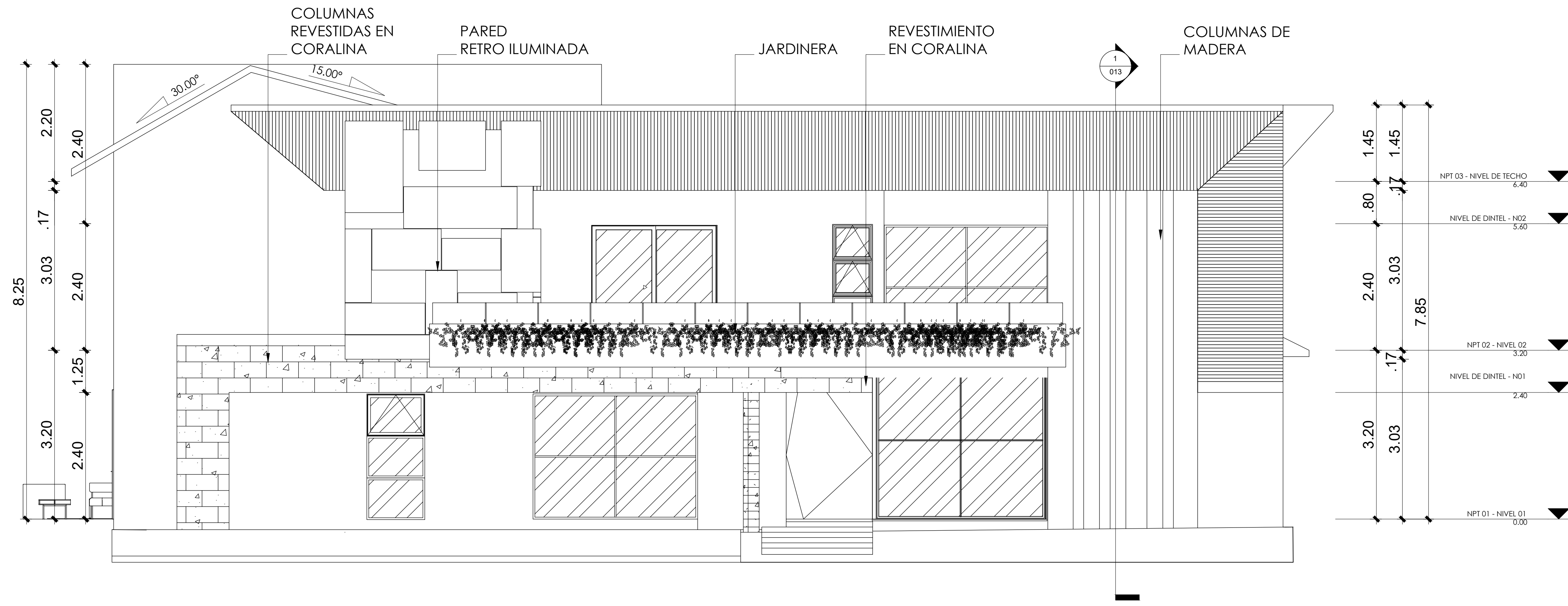
1 ELEVACION FRONTAL 1 : 50
