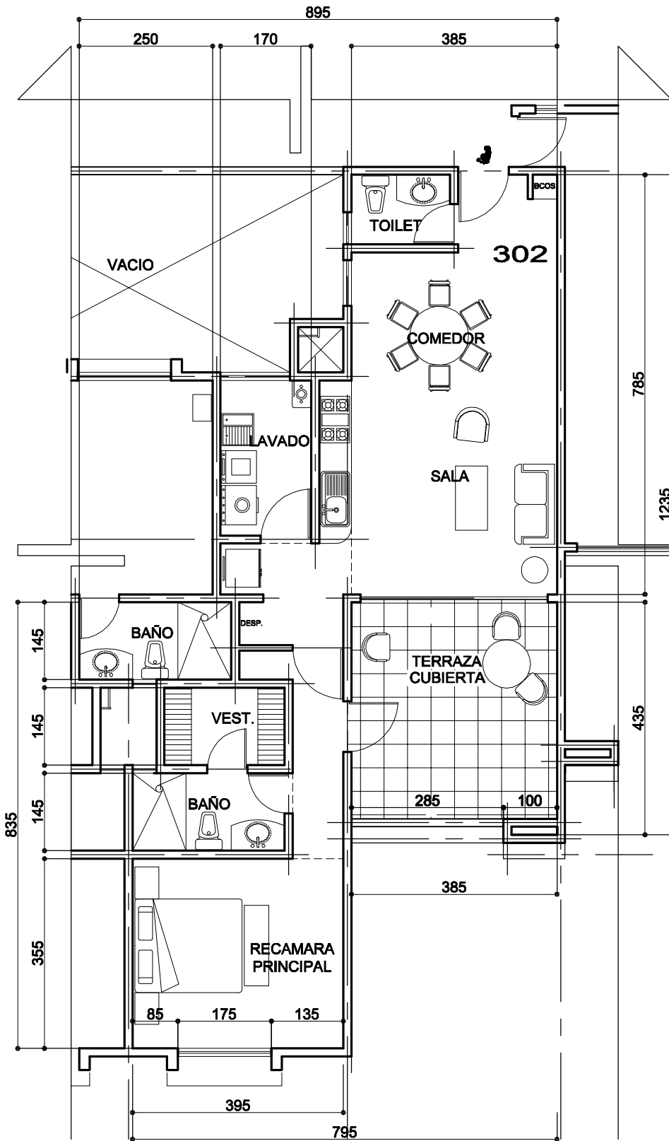
DEPARTAMENTO 3-302 AREA=91.34m 2
