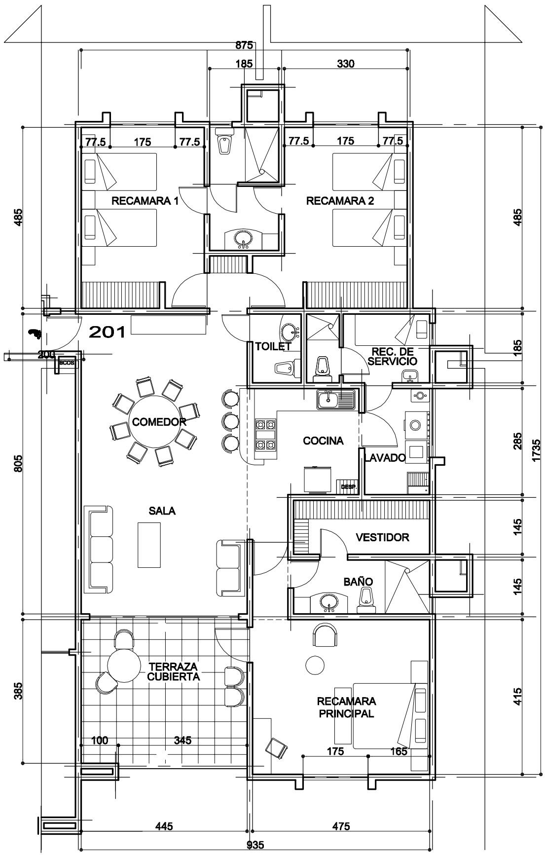
DEPARTAMENTO 3-201 AREA=166.15m 2
