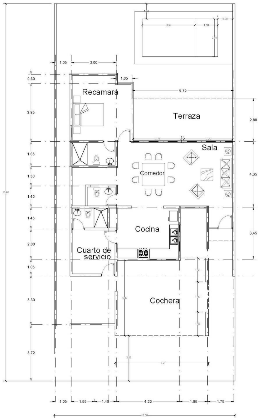
PLANTA ARQUITECTONICA P.B. 149.68 m 2
