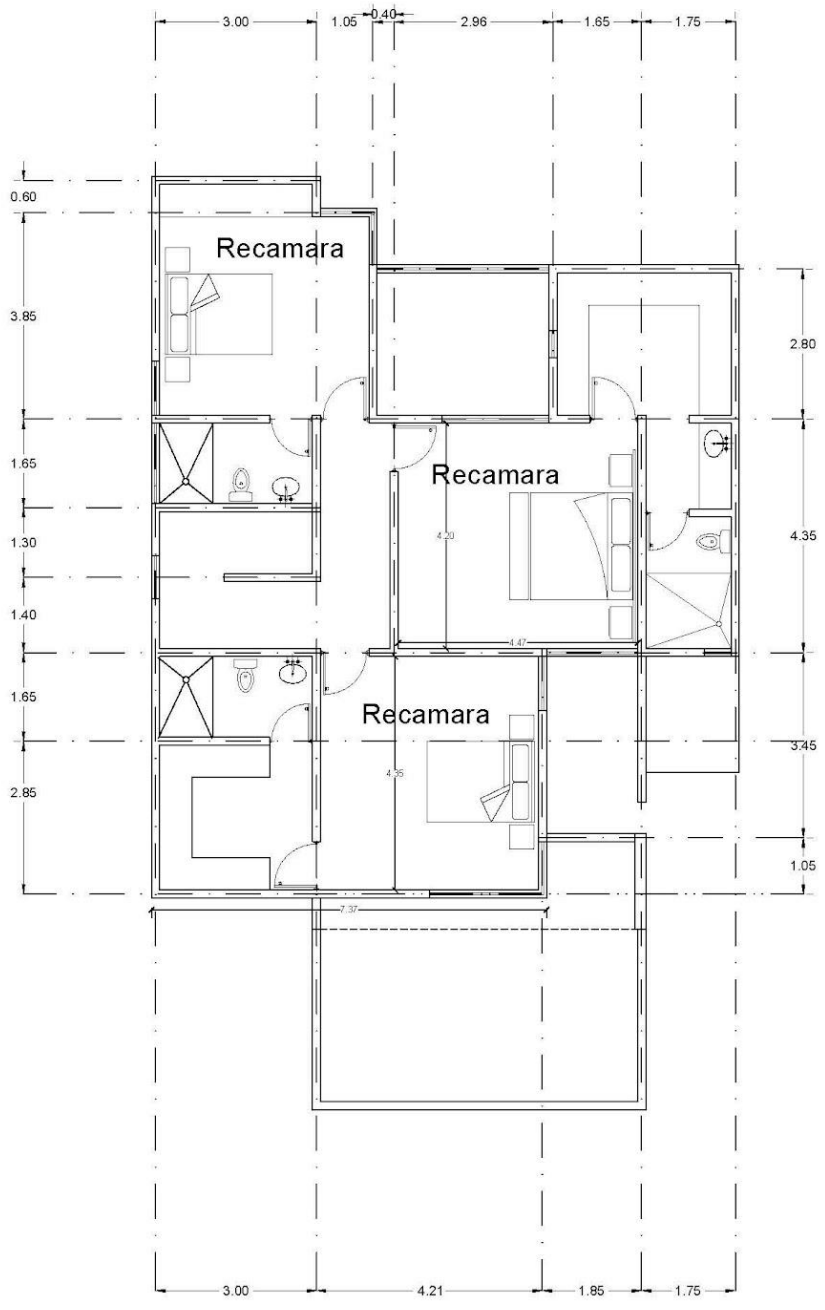
PLANTA ARQUITECTONICA P.A. 116.22 m2
