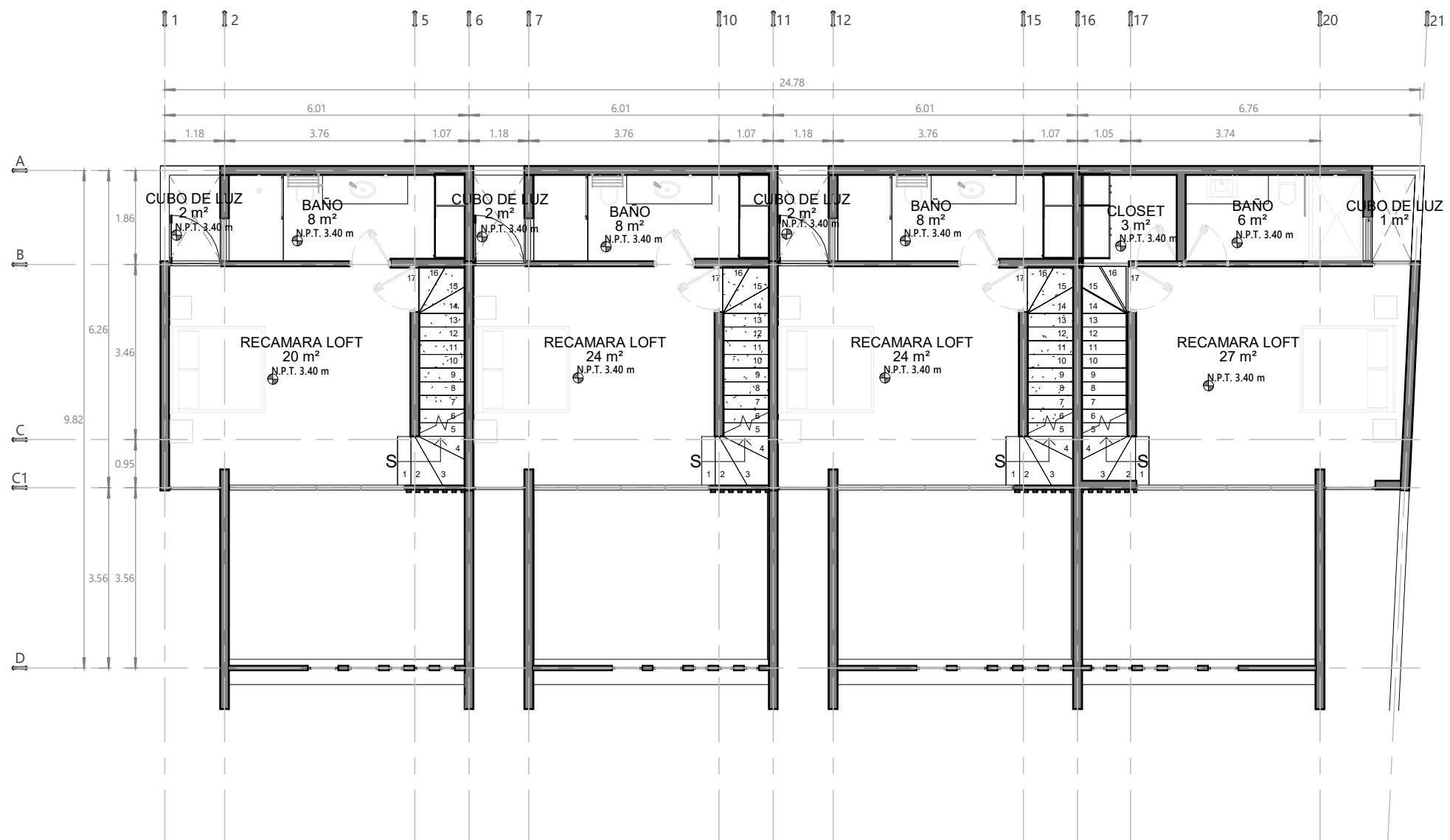
1 | 02.Nivel 1 1 : 100
