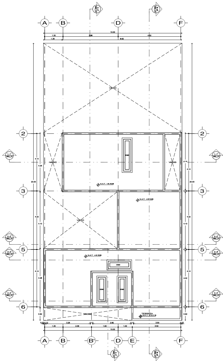
Planta Azotea
