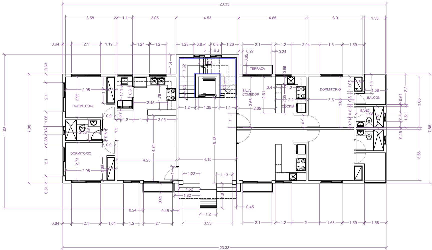
PLANTA DIMENSIONADA 1er NIVEL BLOQUE B ESCALA 1:50
