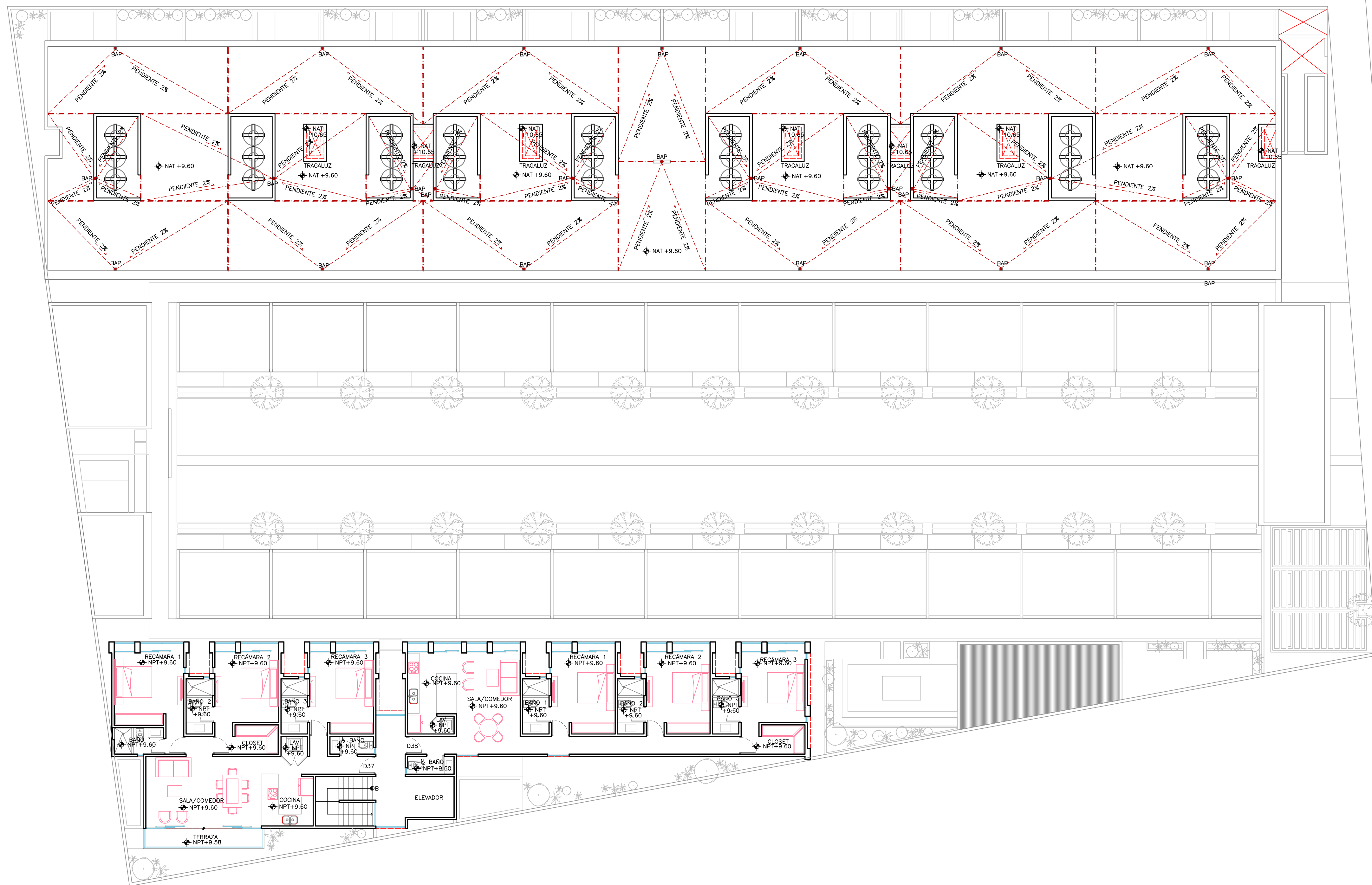
PLANTA TERCER NIVEL
