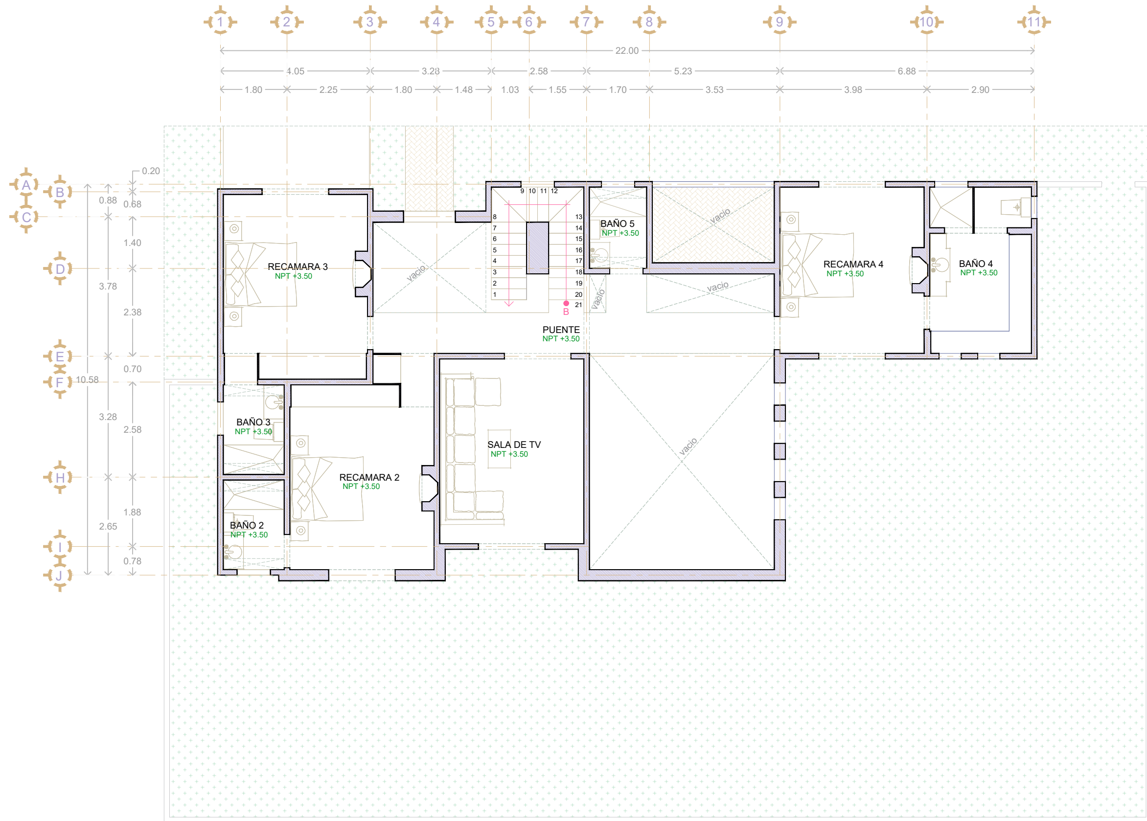
PLANTA ALTA
