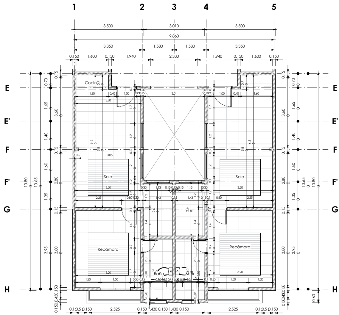
Planta tipo. Depto. 5/9 & 8/12
