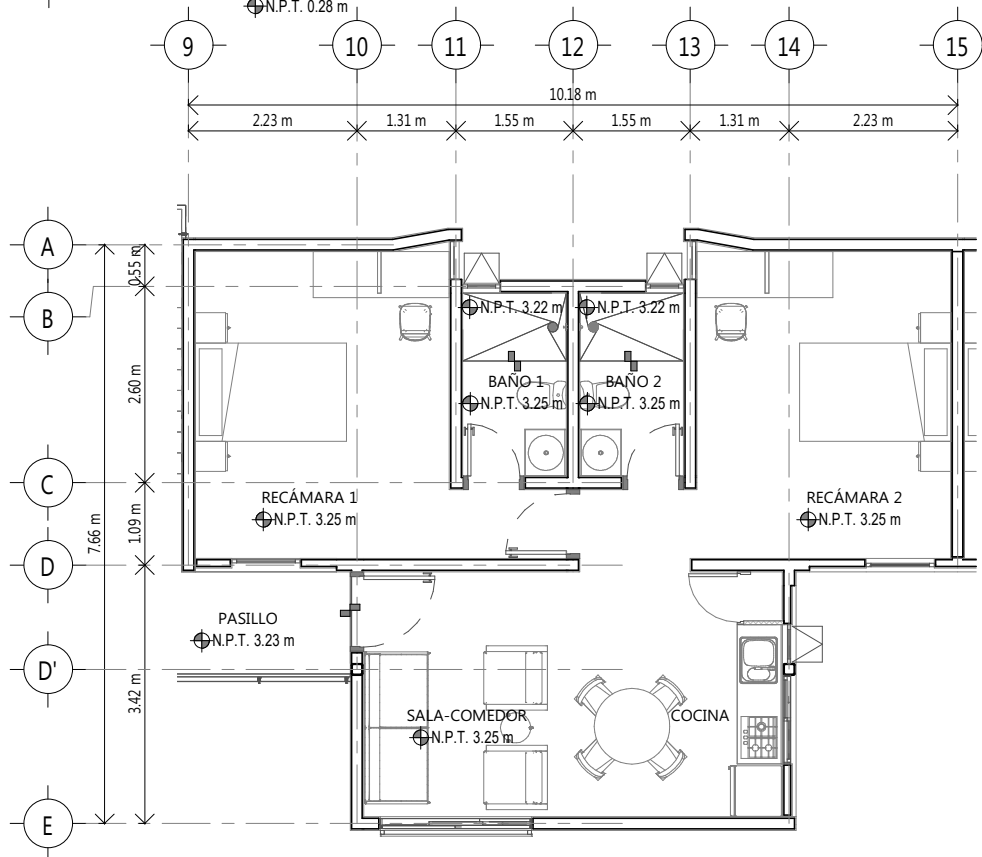
2 Apartamento de 65 m 2 1 : 100
