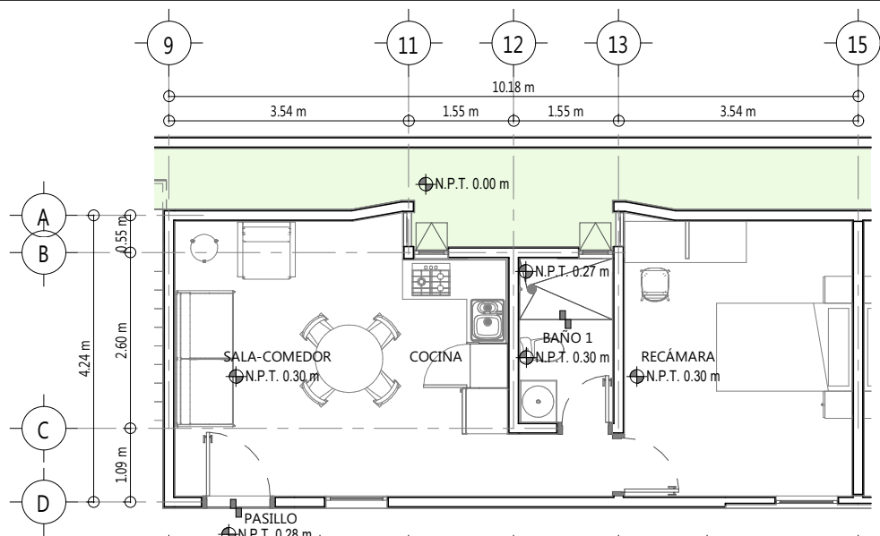
1 Apartamento de 45 m 2 1 : 100
