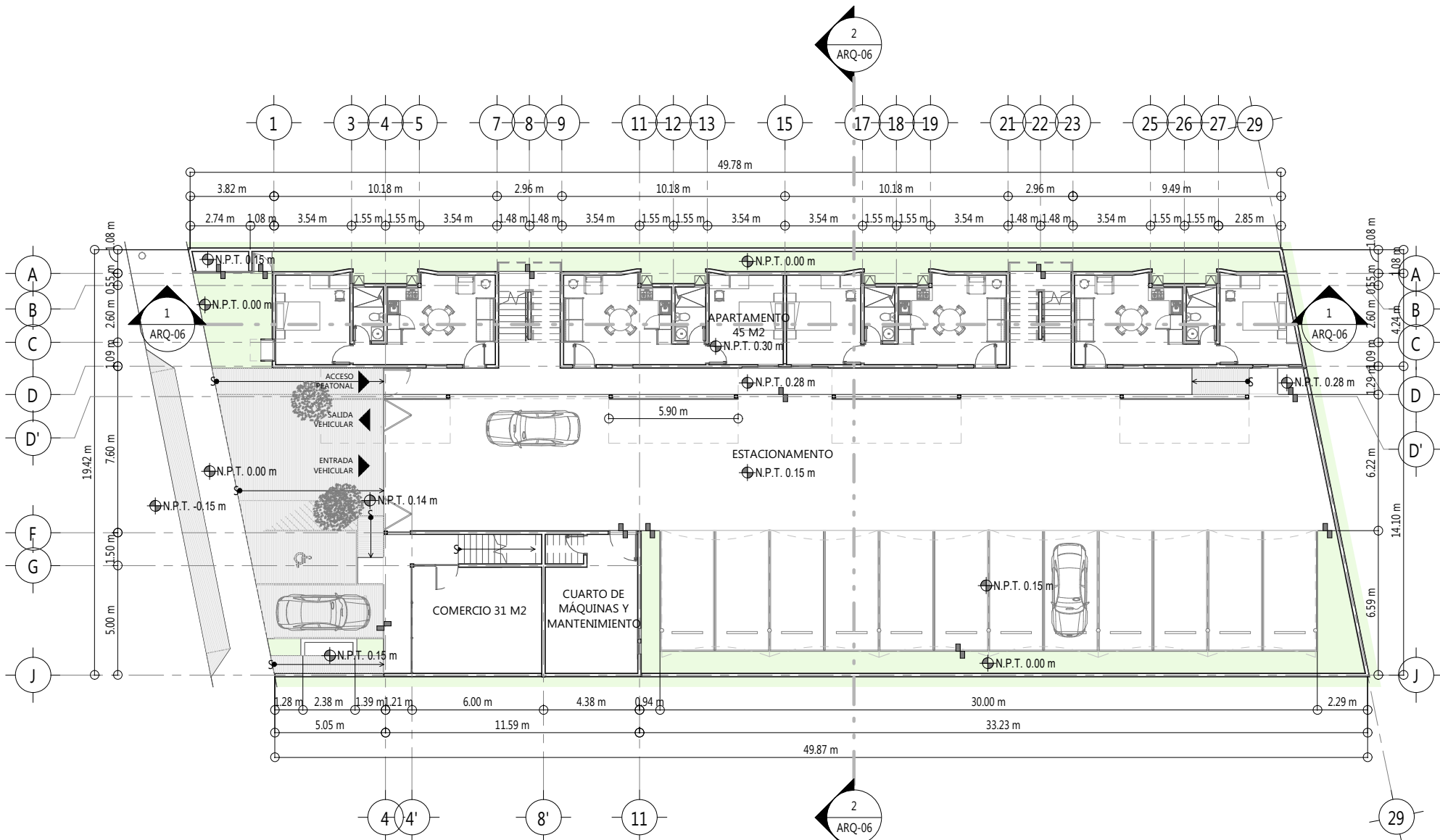
1 Planta Baja 1 : 250
