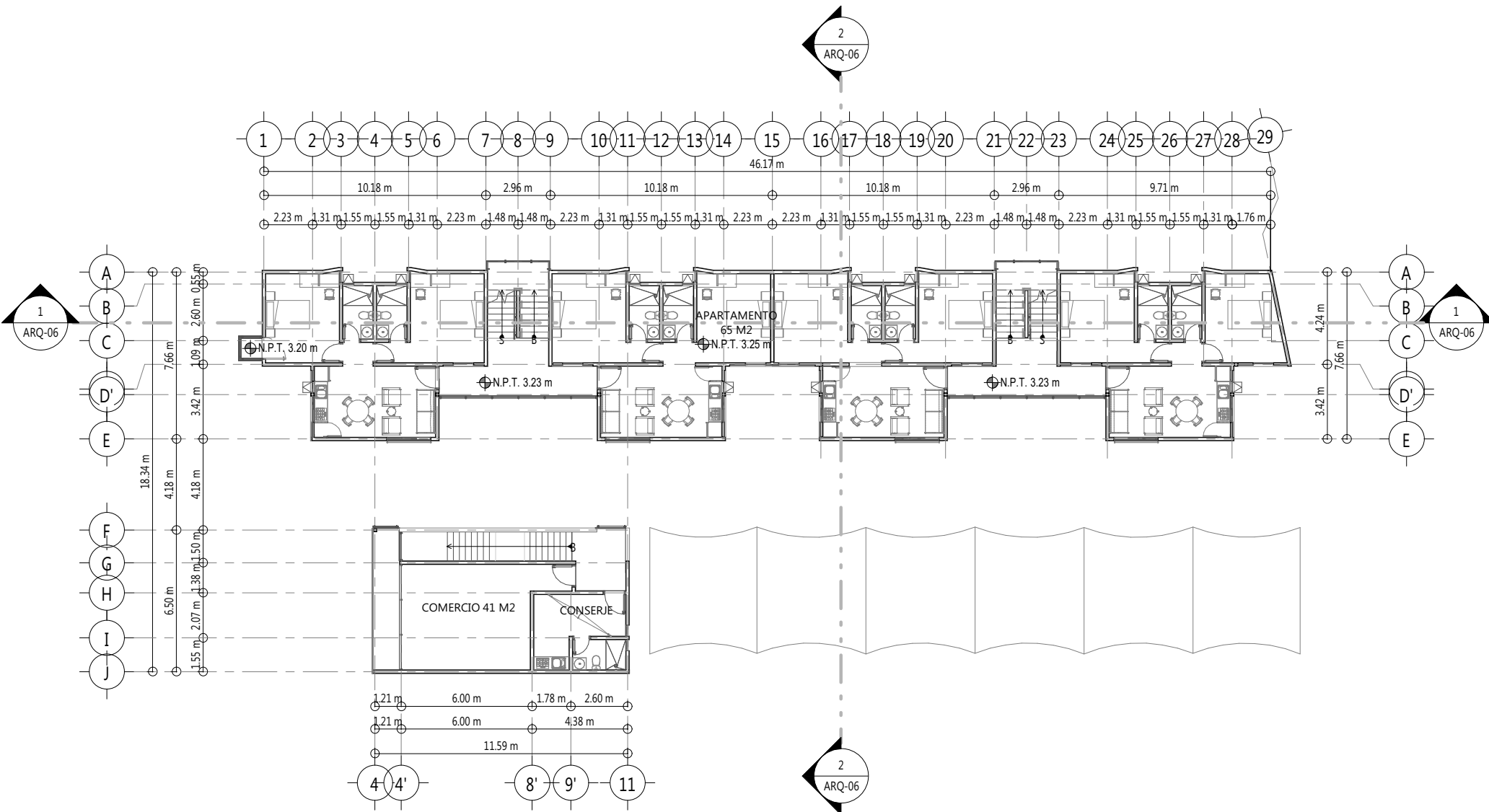
1 Niveles 1-2 1 : 250
