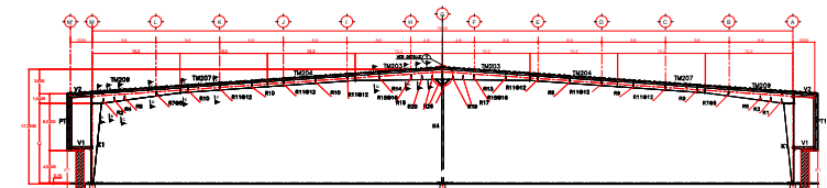
CORTE TRANSVERSAL ELEVACIÓN SOBRE EJES PARES
