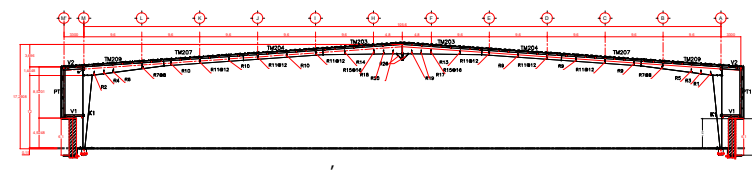
CORTE TRANSVERSAL ELEVACIÓN SOBRE EJES NONES
