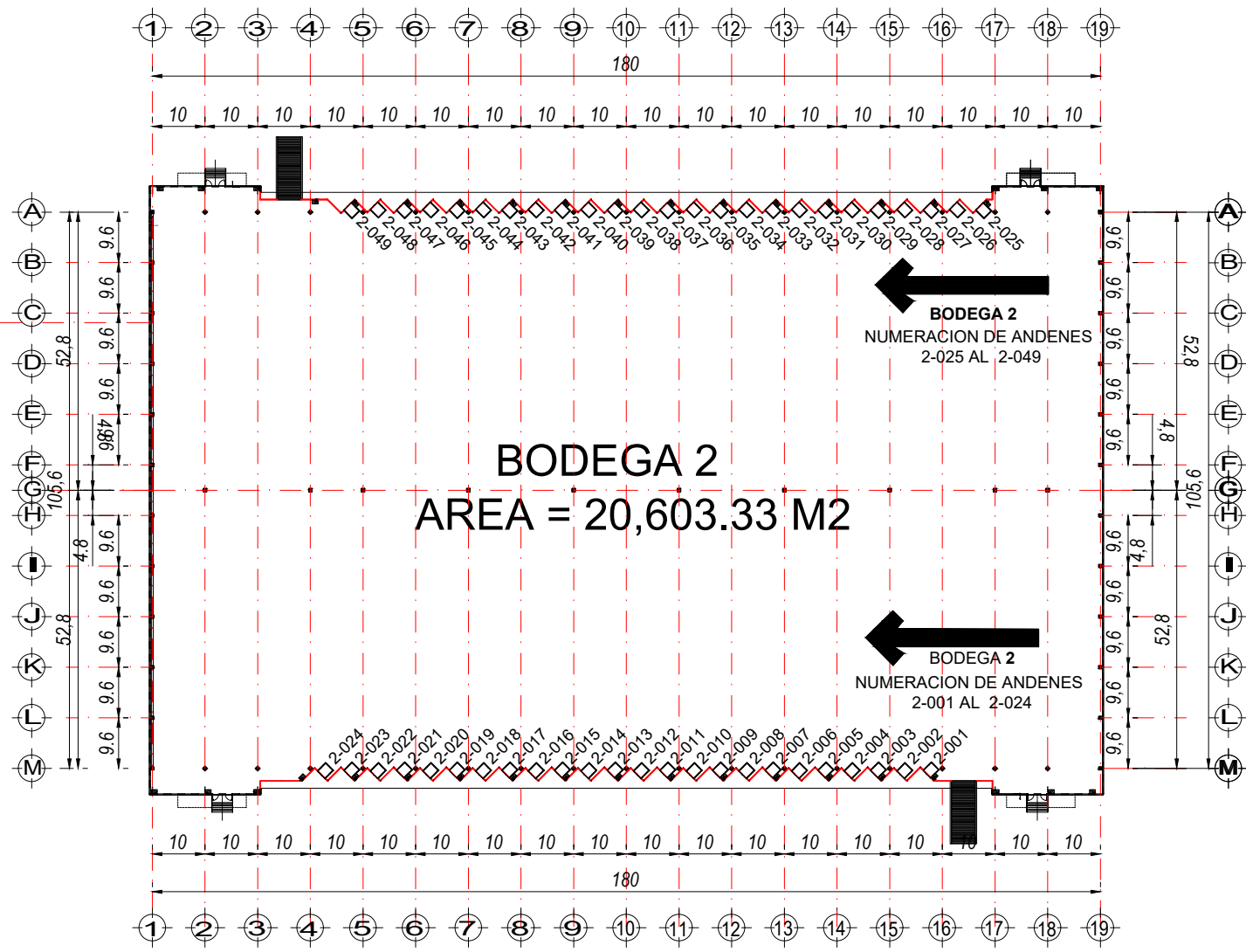
PLANTA ARQUITECTONICA BODEGA 2
