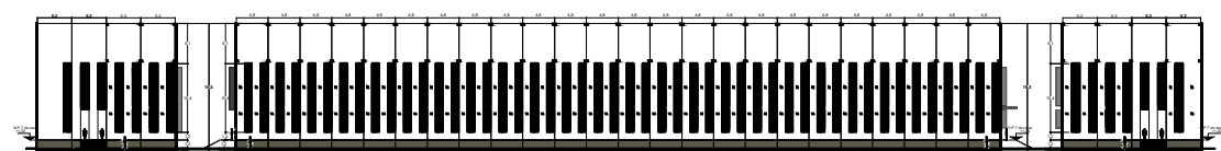
FACHADA MURO CABECERO EJE 1 ( VISTA PONIENTE)
