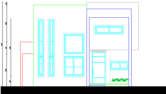
ELEVACION FRONTAL
