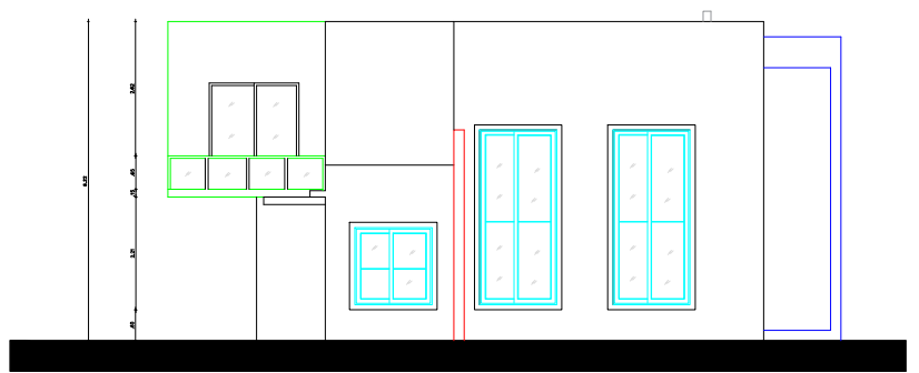
ELEVACION LATERAL IZQUIERDA
