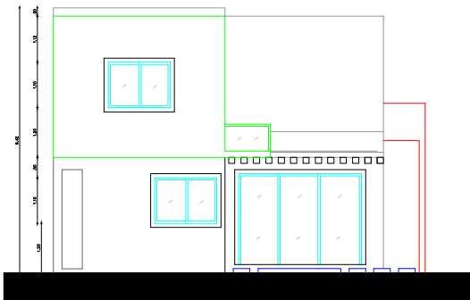
ELEVACION POSTERIOR
