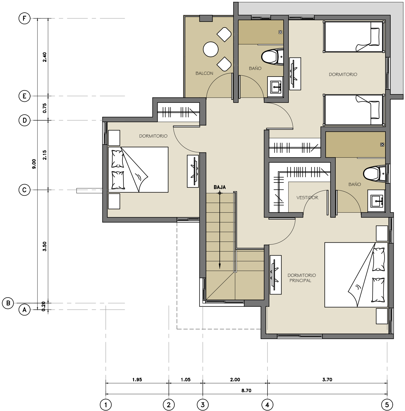
2 PLANTA ARQ. AMUEBLADA 2do. NIVEL A--- ESCALA 1:---
