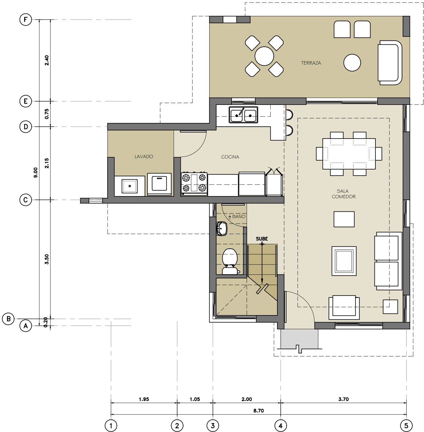
1 PLANTA ARQ. AMUEBLADA 1er. NIVEL A ESCALA 1:--
