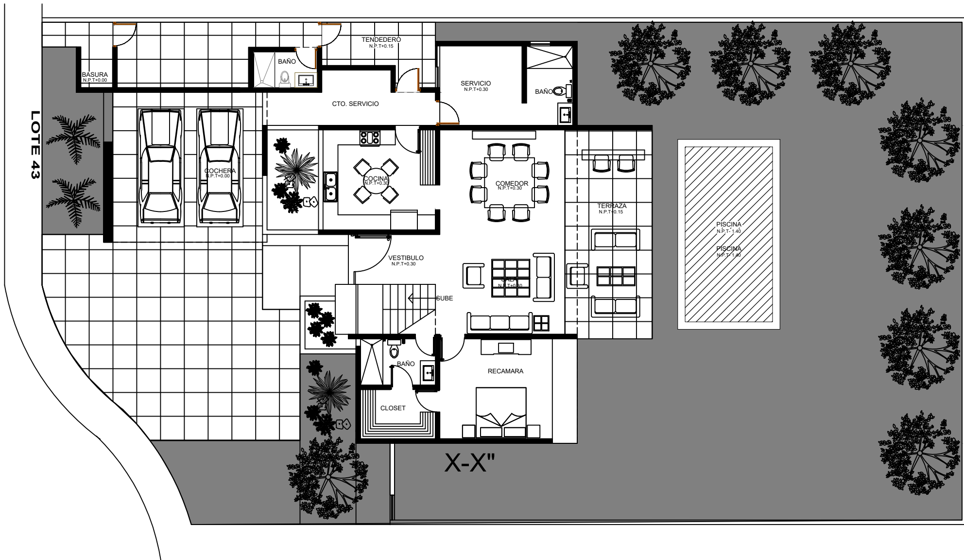
PLANTA ARQUITECTONICA BAJA
