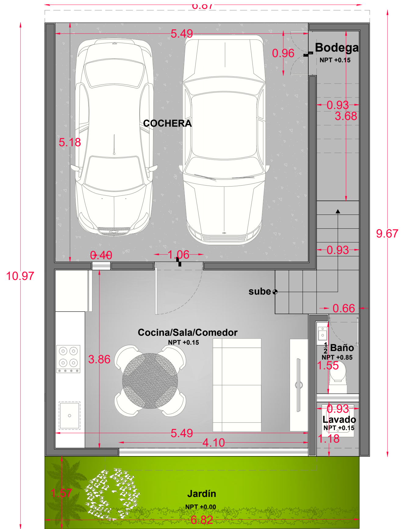
Planta Baja
