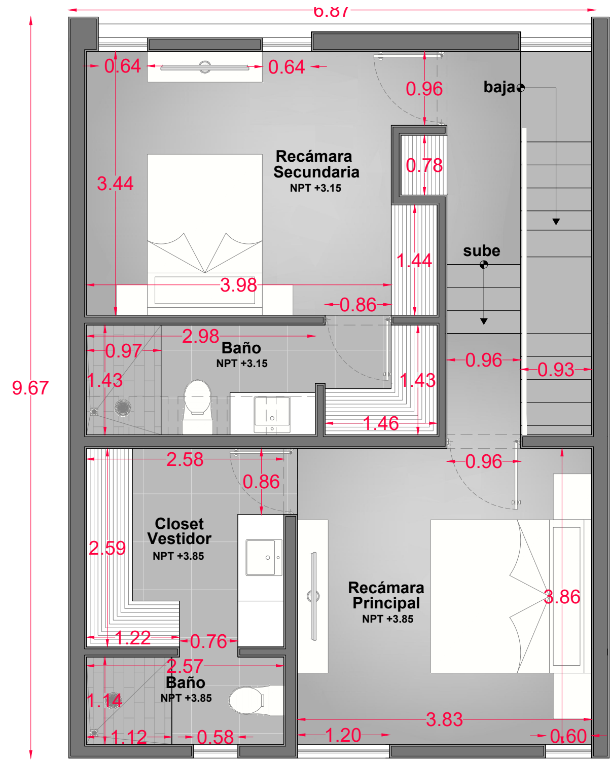
Planta Alta
