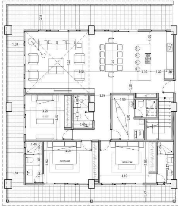
PLANTA BAJA
