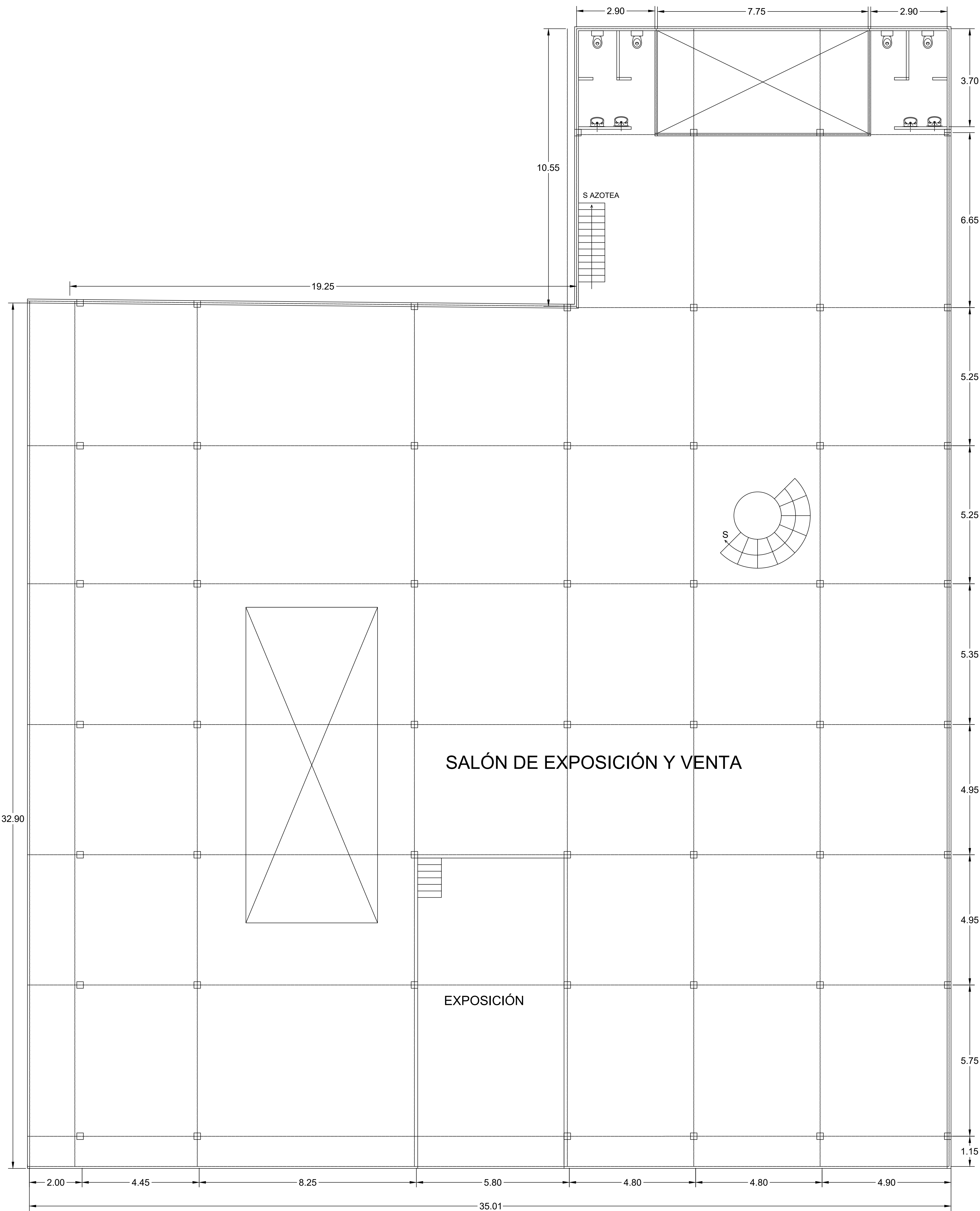
PLANTA 1ER Y 2DO NIVEL
