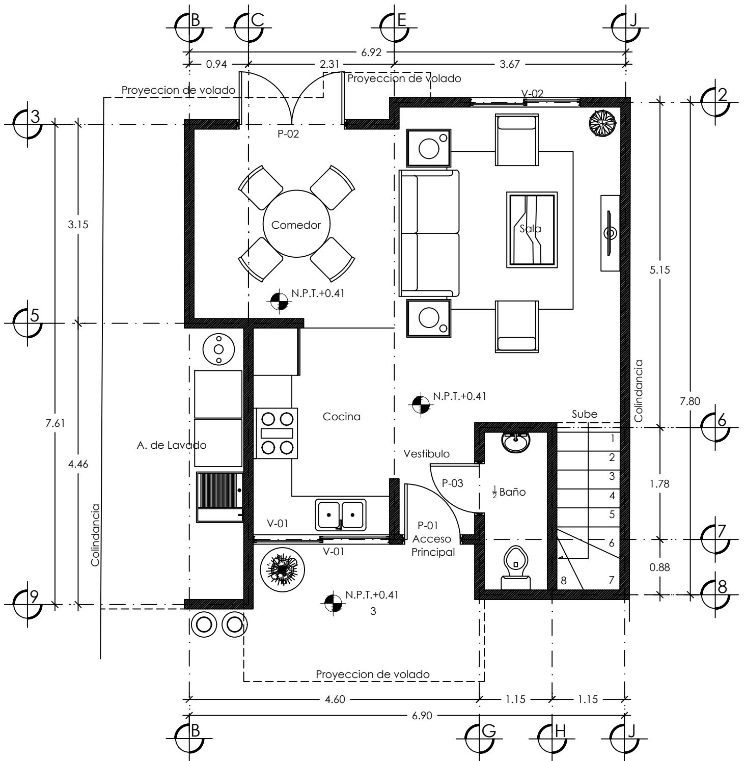
PLANTA ARQUITECTONICA BAJA AREA= 62.10 m2
