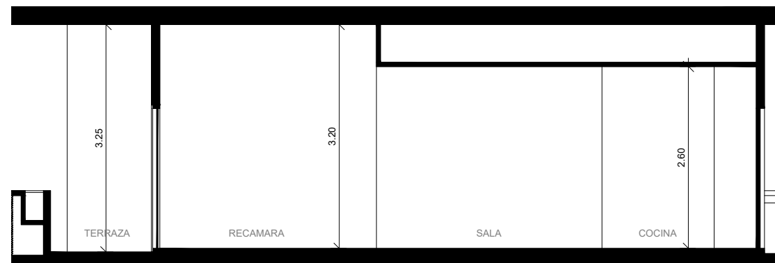
SECCION A-A' ESC. 1:75
