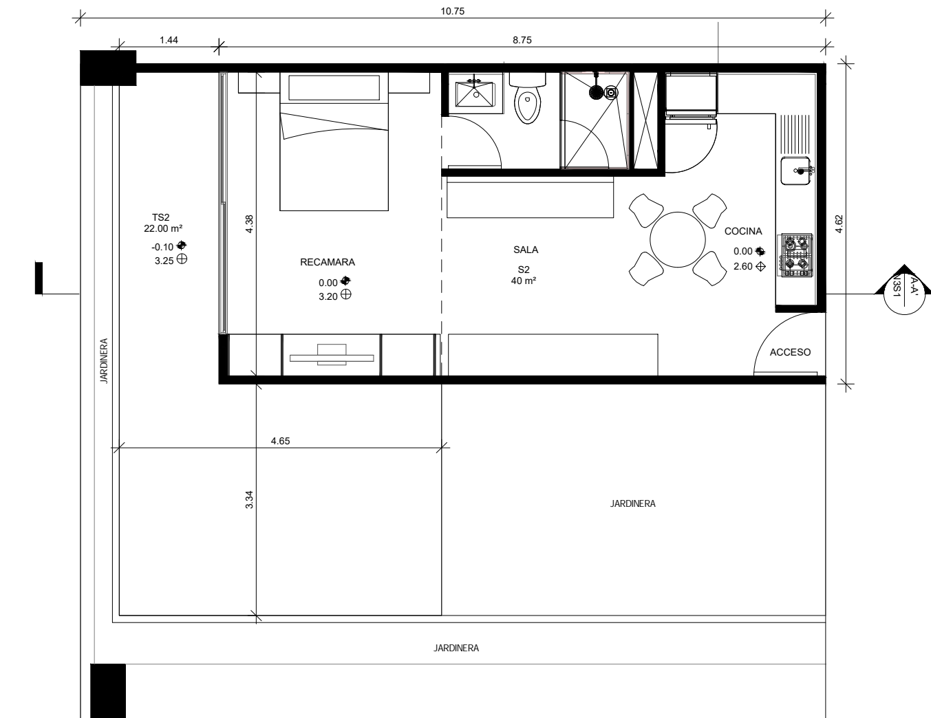
PLANTA ESC. 1:75
