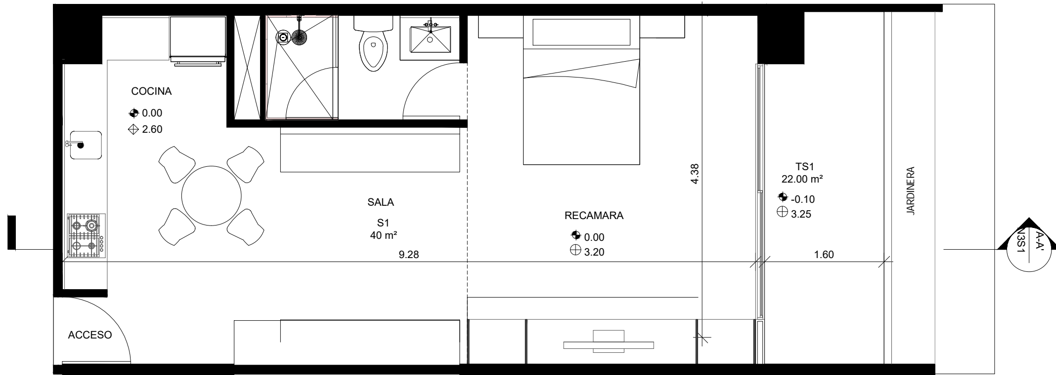
PLANTA ESC. 1:50
