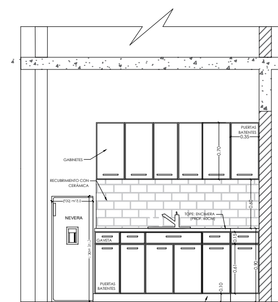
ELEVACIÓN - VISTA 1
