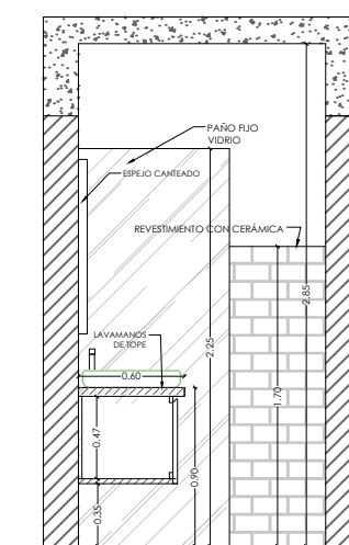
ELEVACIÓN - VISTA 2
