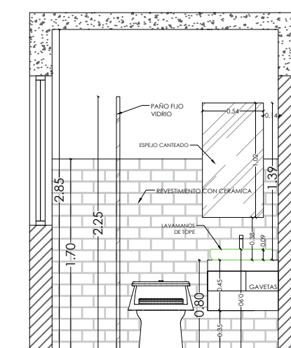
ELEVACIÓN - VISTA 1
