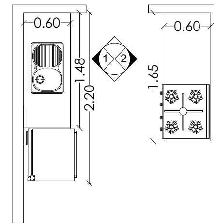
PLANTA COCINA TIPO A
