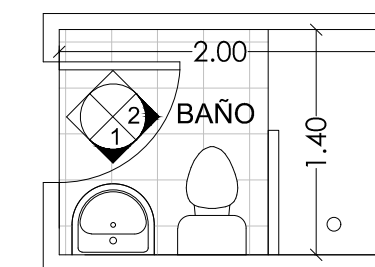
PLANTA BAÑO TIPO A
