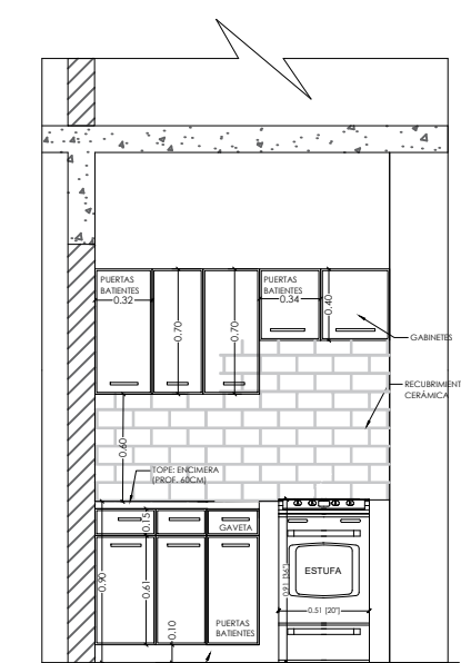
ELEVACIÓN - VISTA 2
