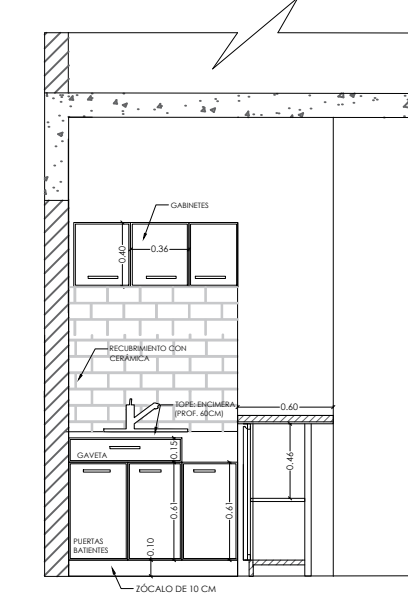
ELEVACIÓN - VISTA 1
