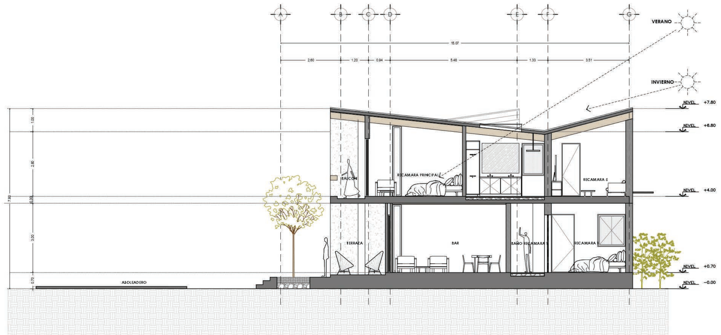
CORTE 3-3'
