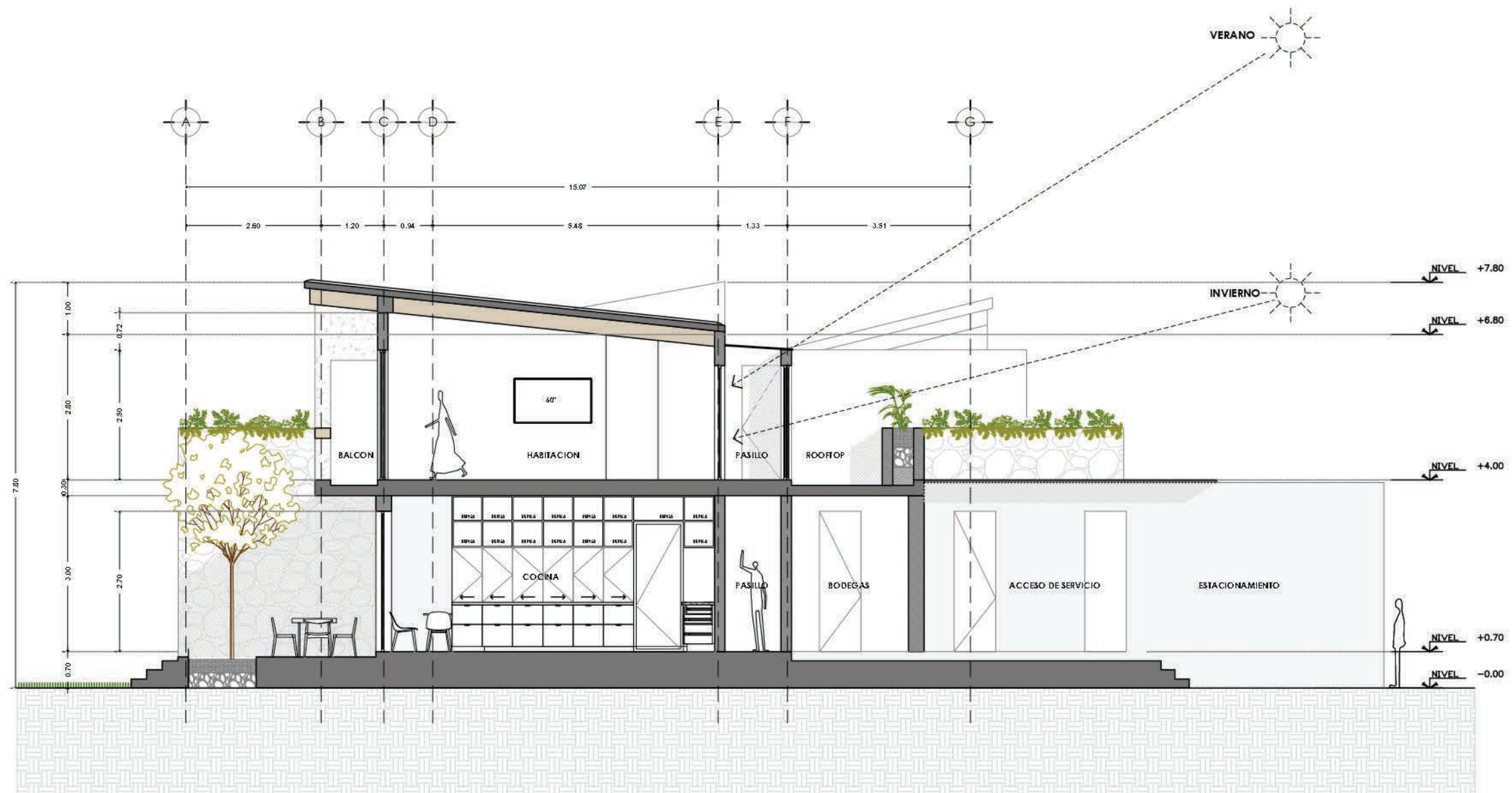
CORTE 6-6'
