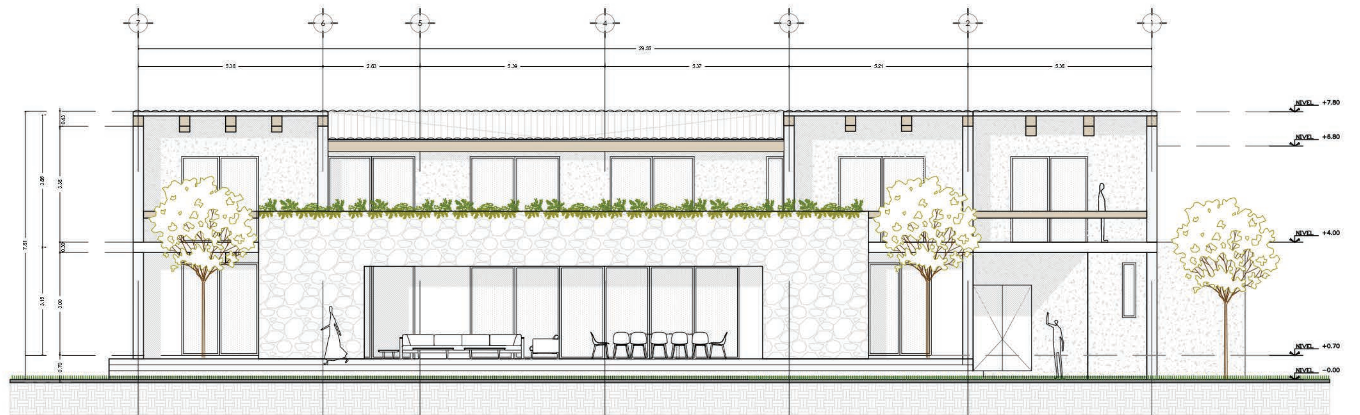
FACHADA POSTERIOR
