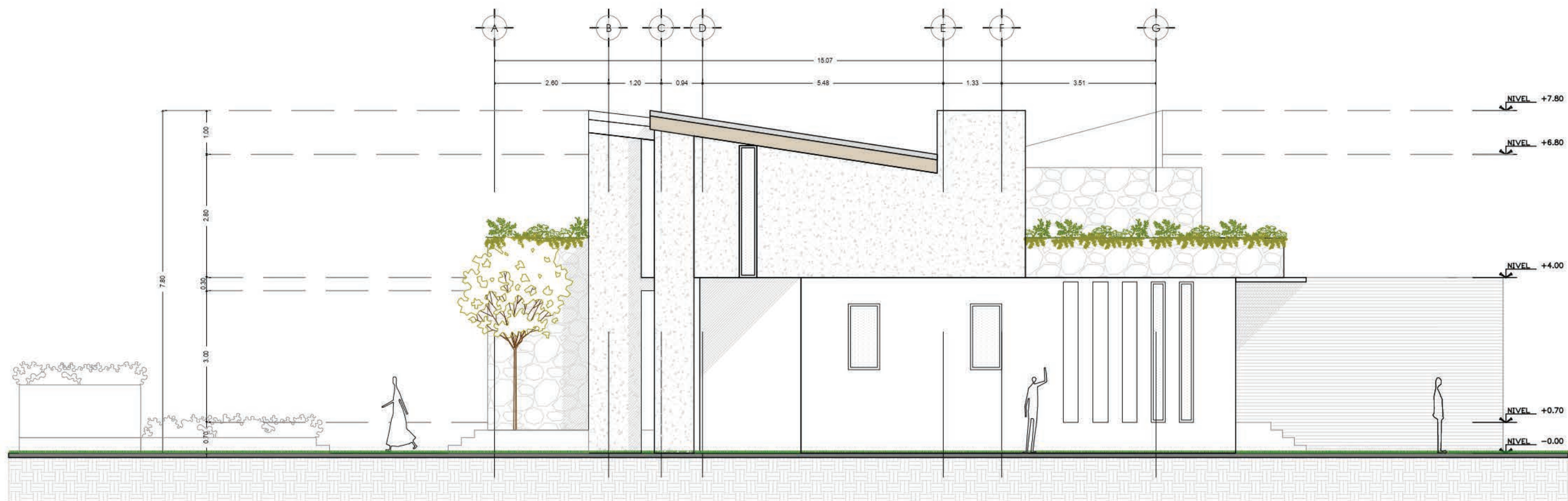
FACHADA LATERAL 2
