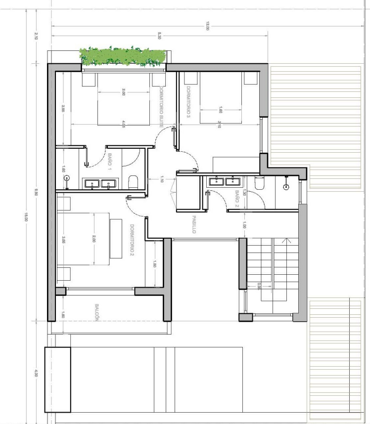
Planta Nivel 2
