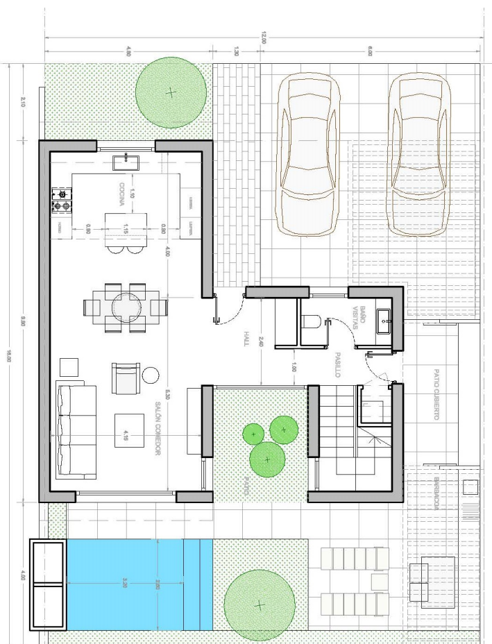
Planta Nivel 1
