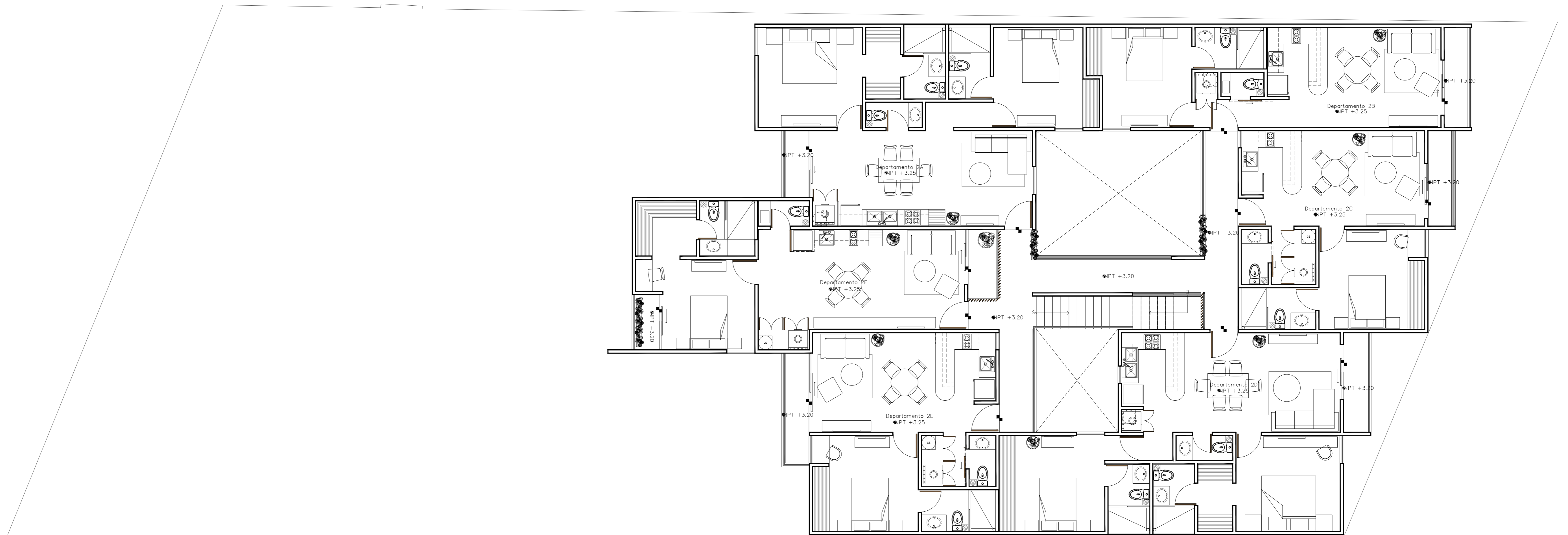
PLANTA PRIMER NIVEL
