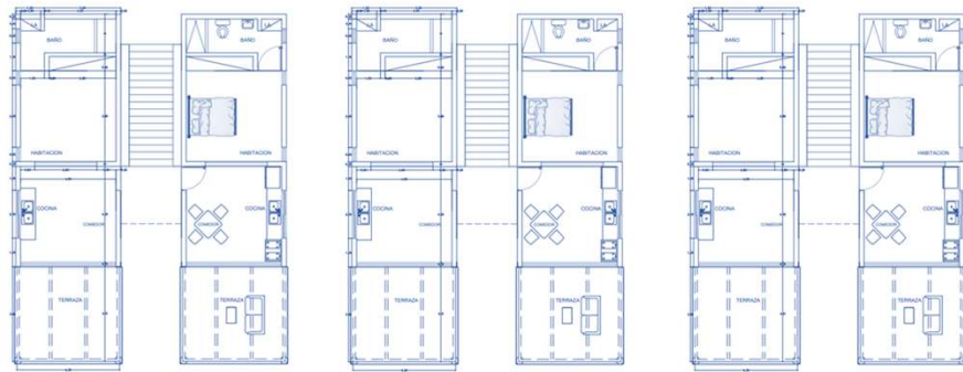
PLANTA DIMENSIONADA SEGUNDO NIVEL
