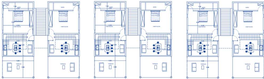
PLANTA ARQUITECTONICA SEGUNDO NIVEL
