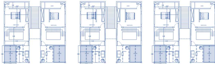
PLANTA ARQUITECTONICA TERCER NIVEL
