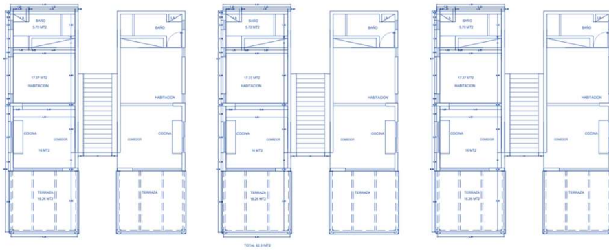
PLANTA DIMENSIONADA PRIMER NIVEL
