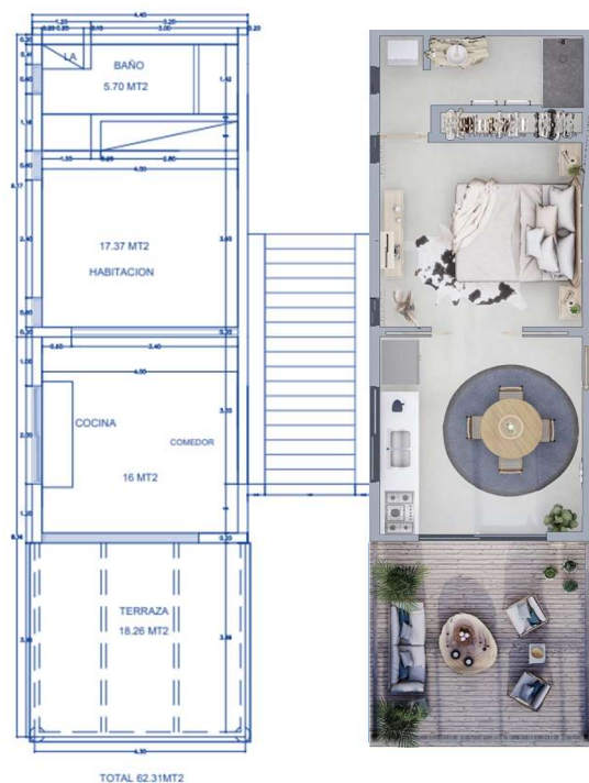
PLANTA DIMENSIONADA PRIMER NIVEL
