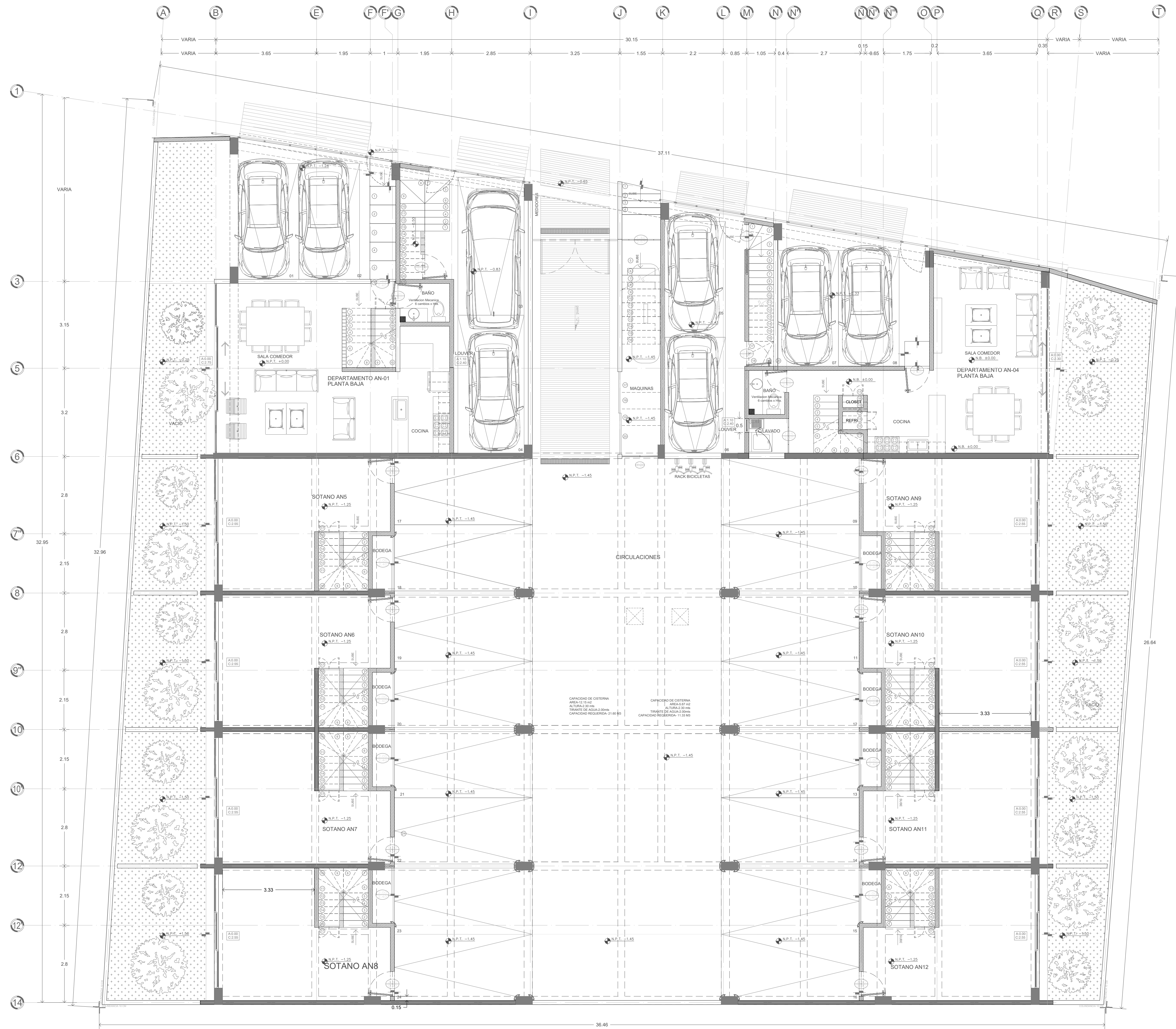
01 PLANTA DE SEMI SOTANO 1:75
