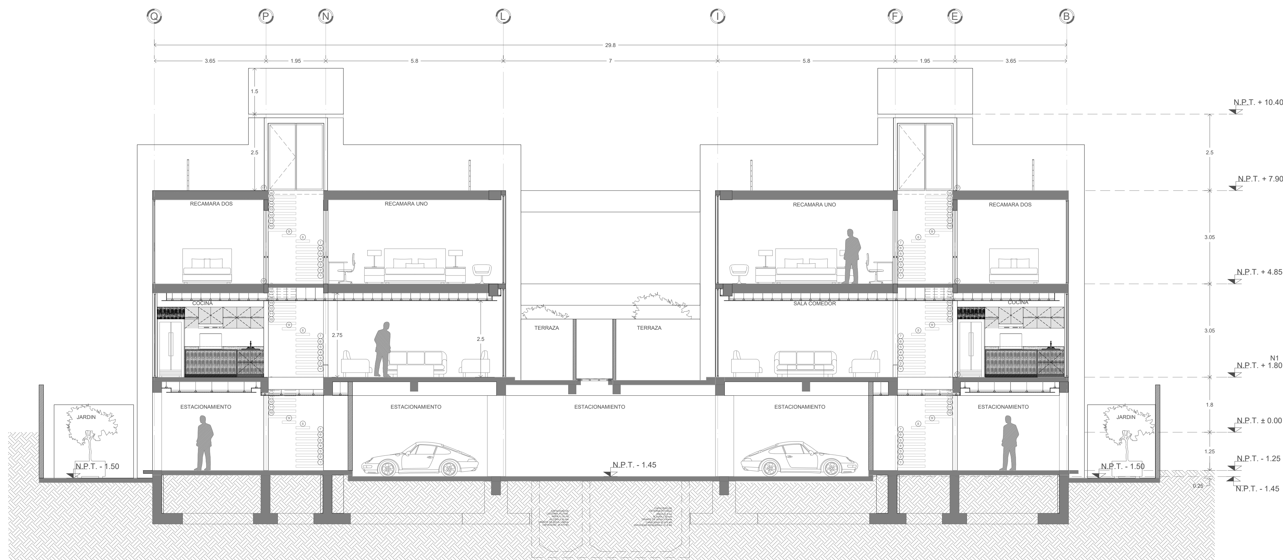
02 CORTE TRANSVERSAL F-F 1:75
