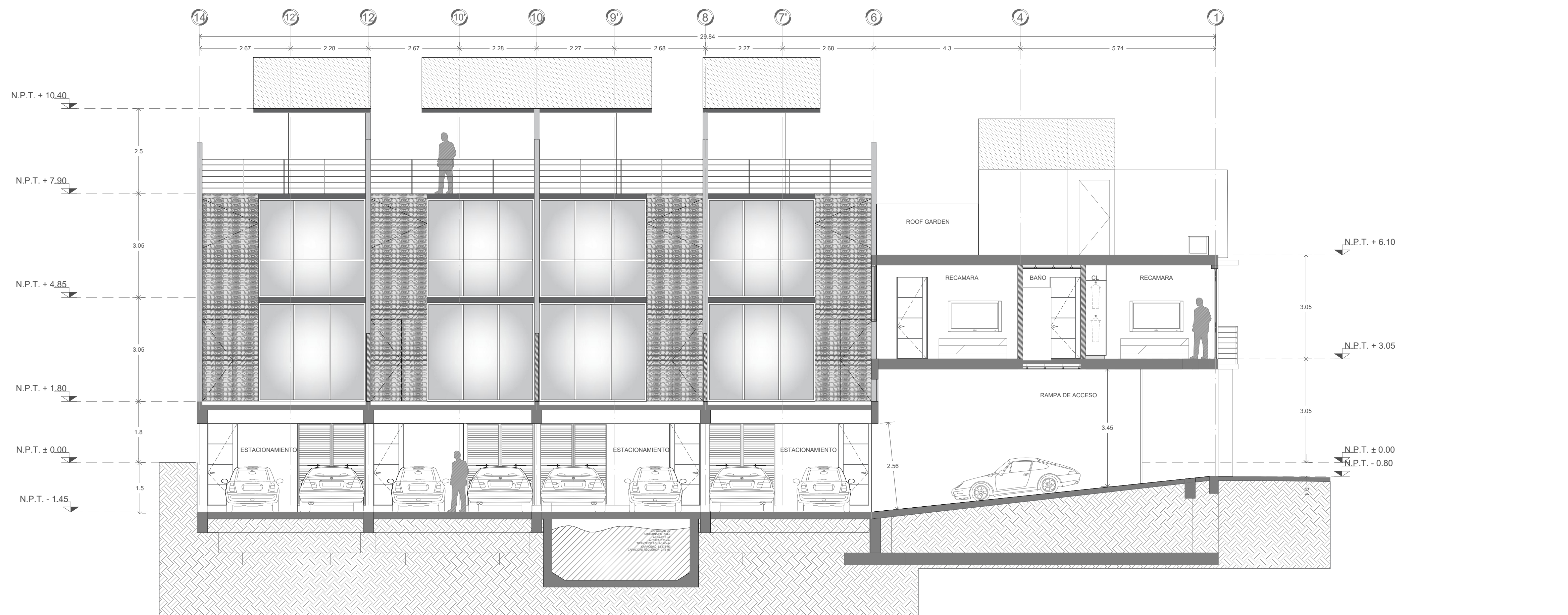
CORTE LONGITUDINAL A-A 1:75
