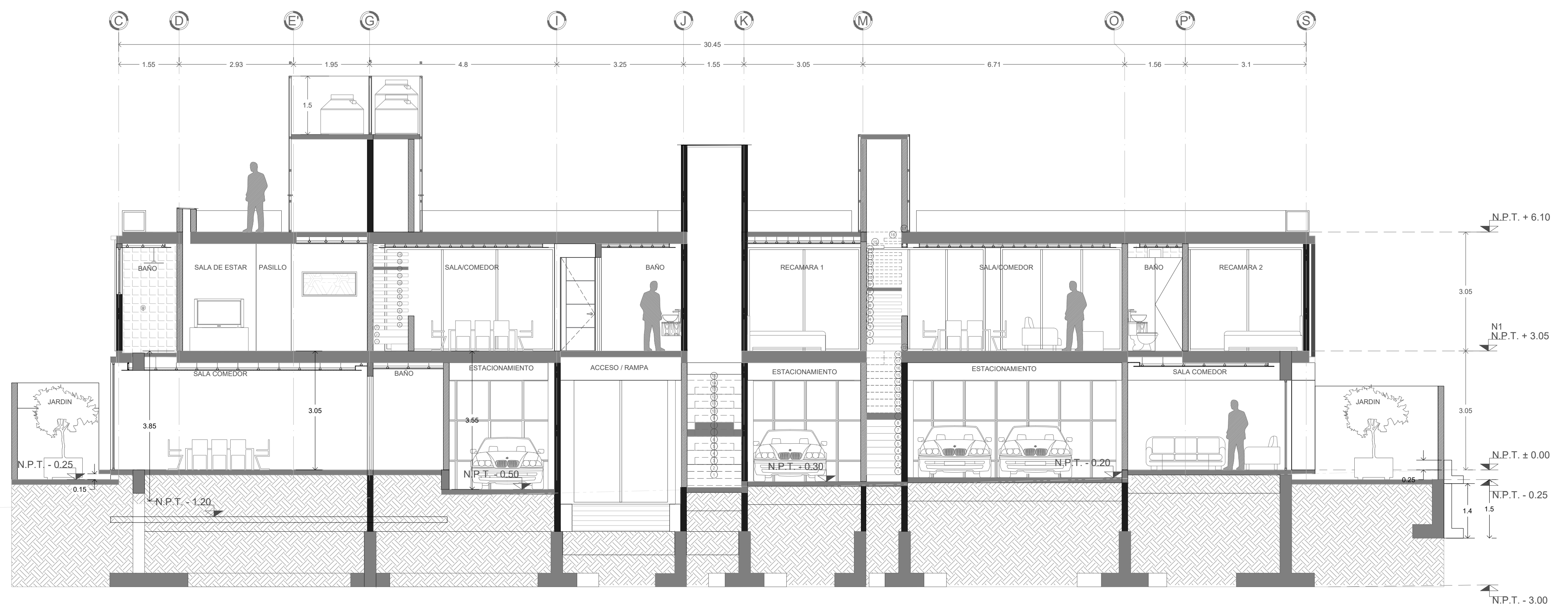
01 CORTE TRANSVERSAL E-E 1:75
