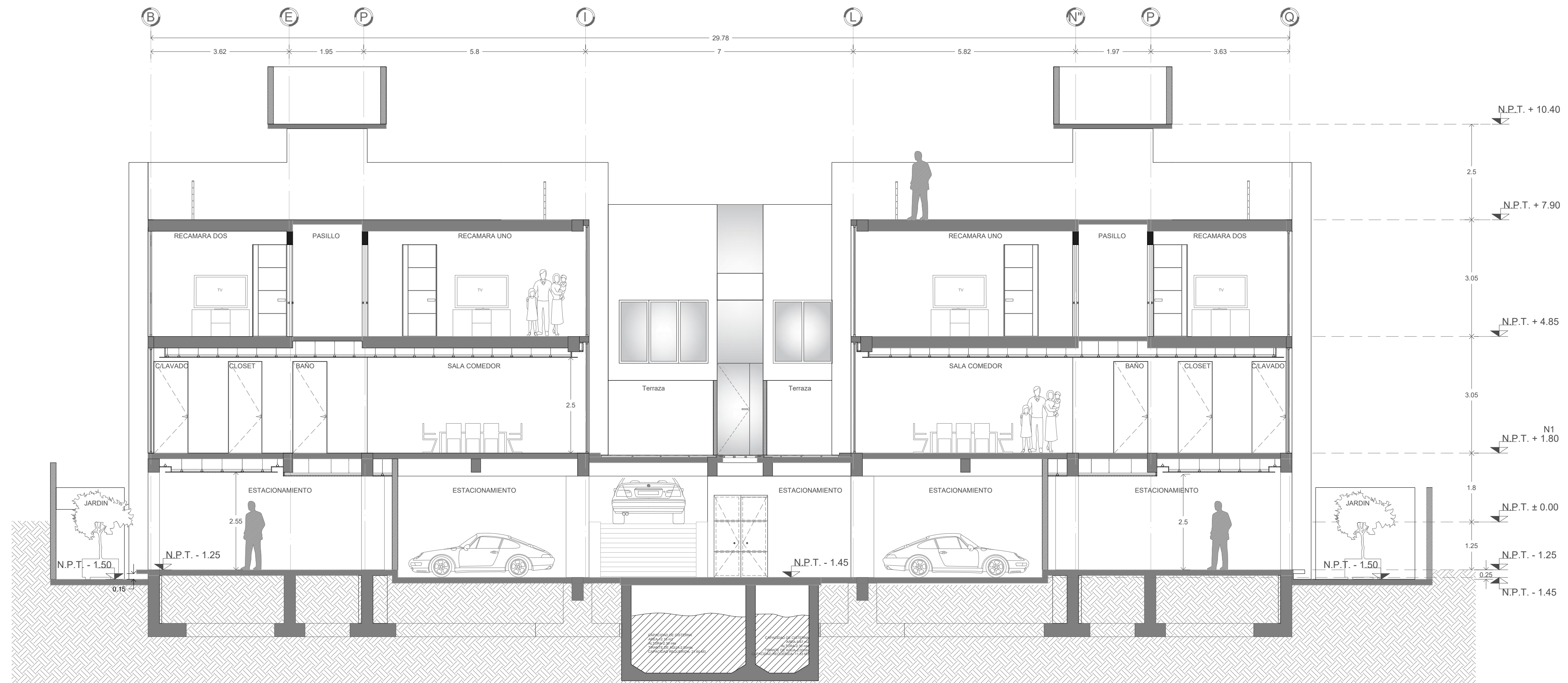
01 CORTE TRANSVERSAL G-G 1:75
