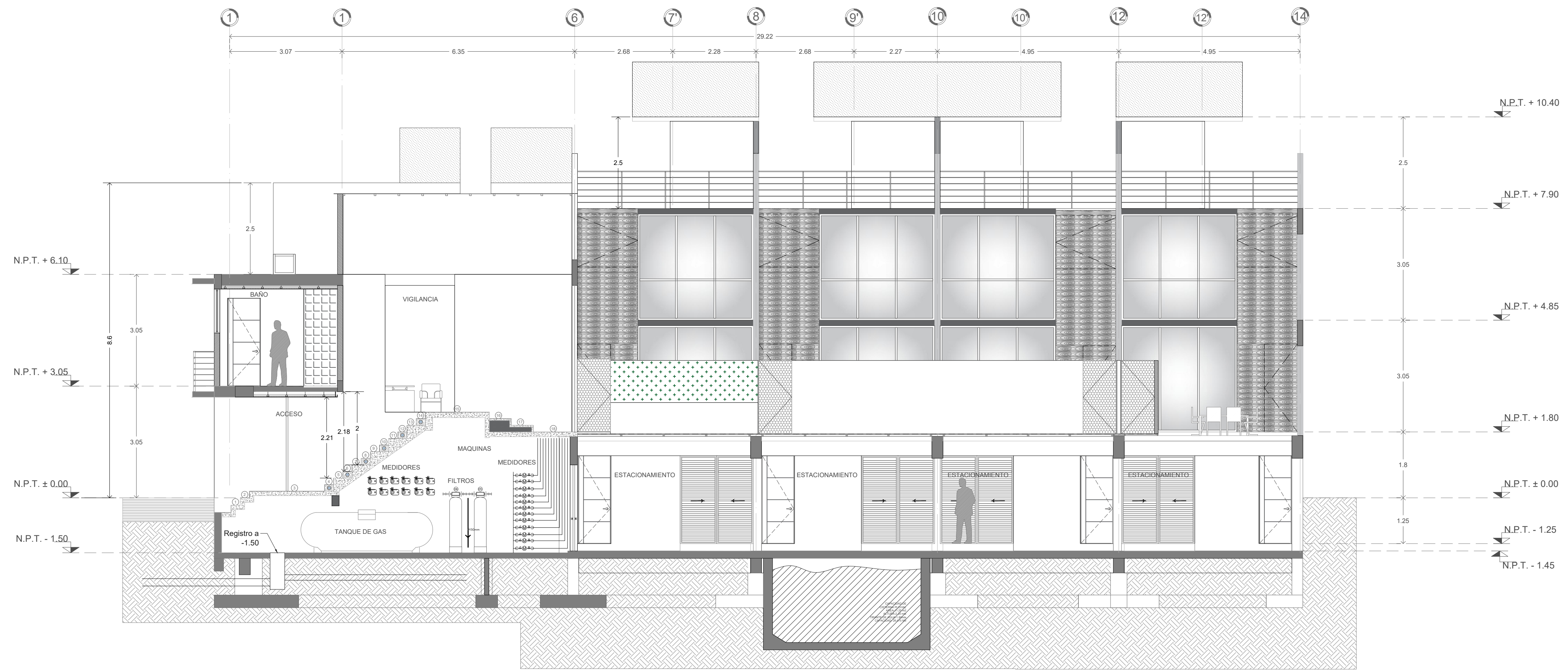
CORTE LONGITUDINAL C-C 1:75
