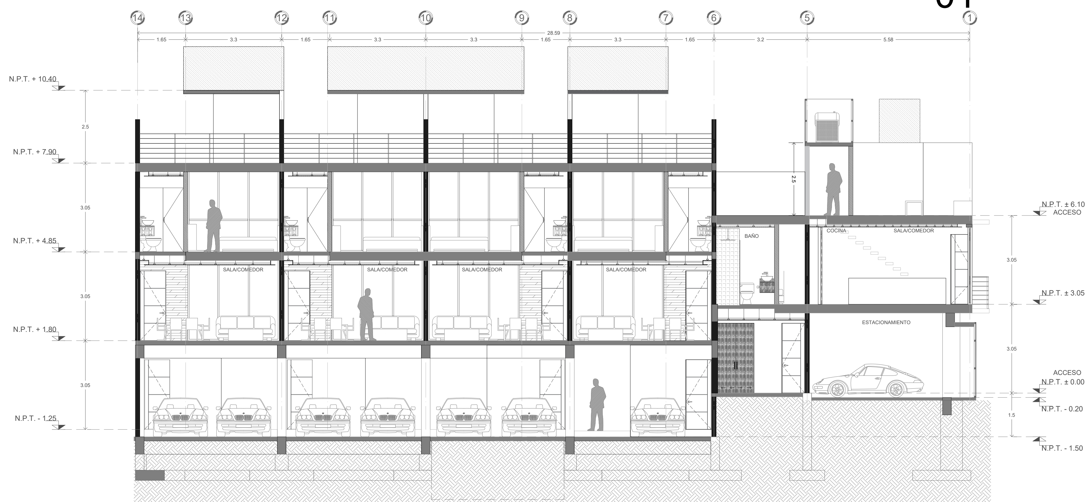
CORTE LONGITUDINAL D-D 1:75
